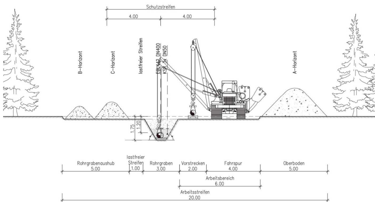
Abbildung 2: Typenplan Arbeitsstreifen eingeschränkt
