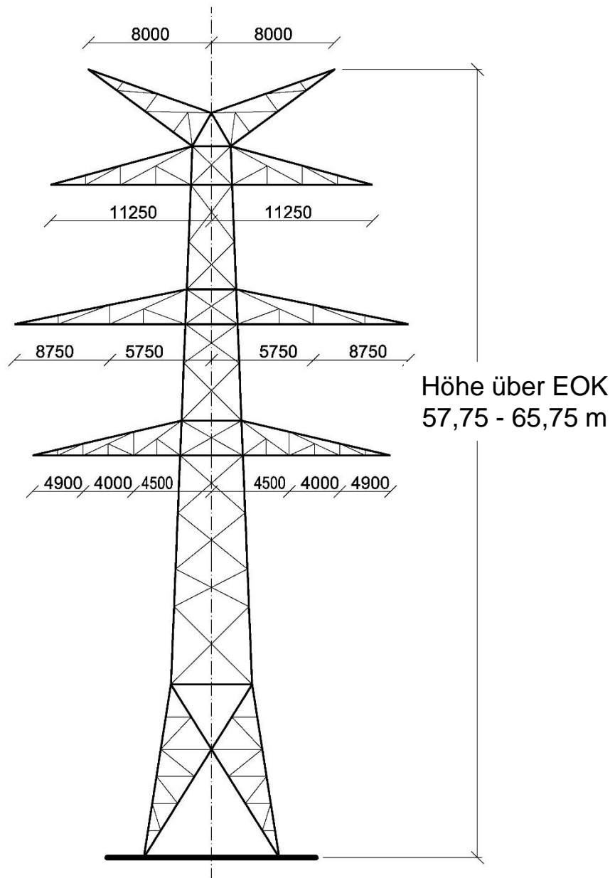
Schemazeichnung (ohne Maßstab) Maßangaben in Millimeter
