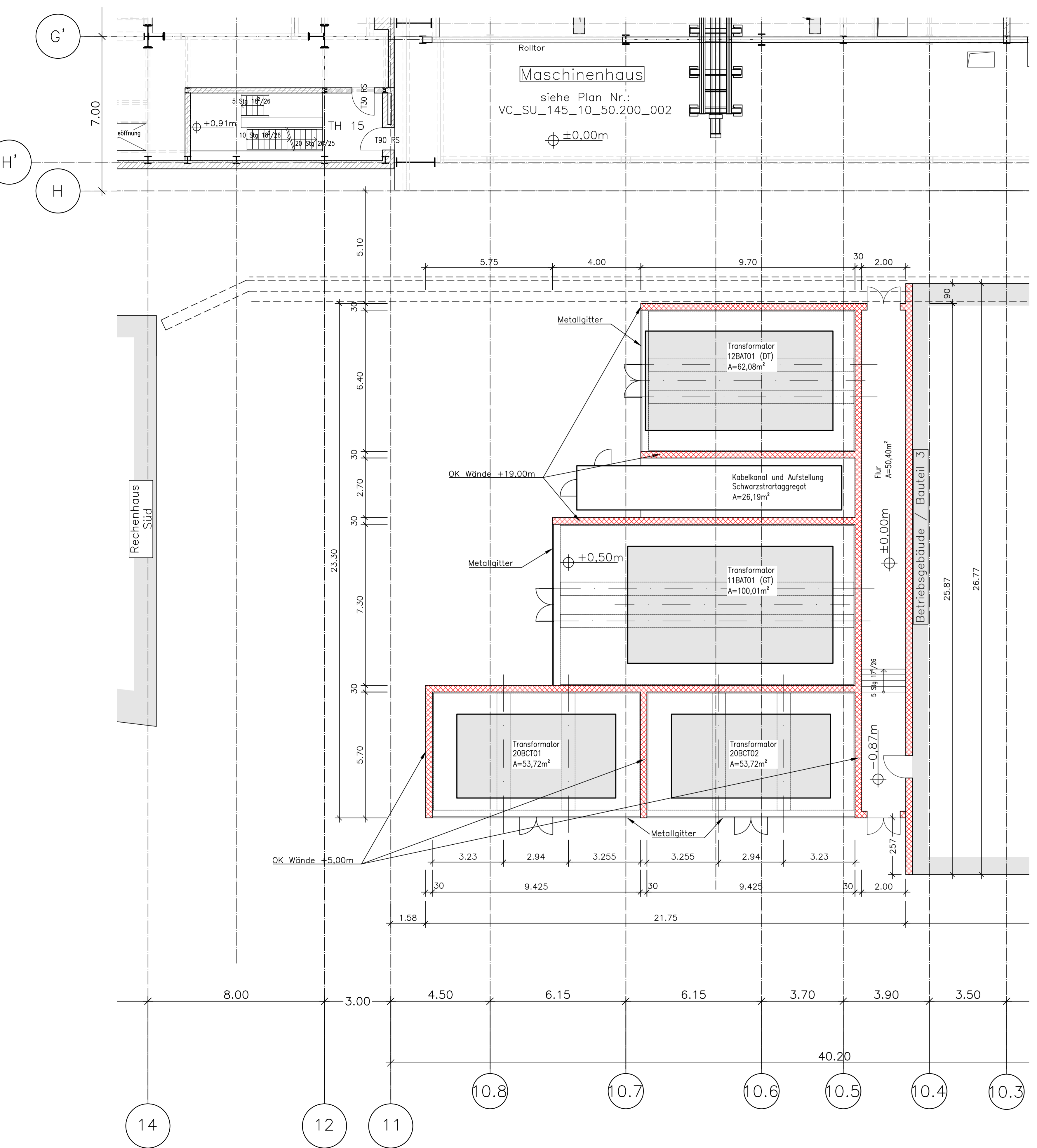
Grundriss ±0,00 (Trafos) M 1:100
