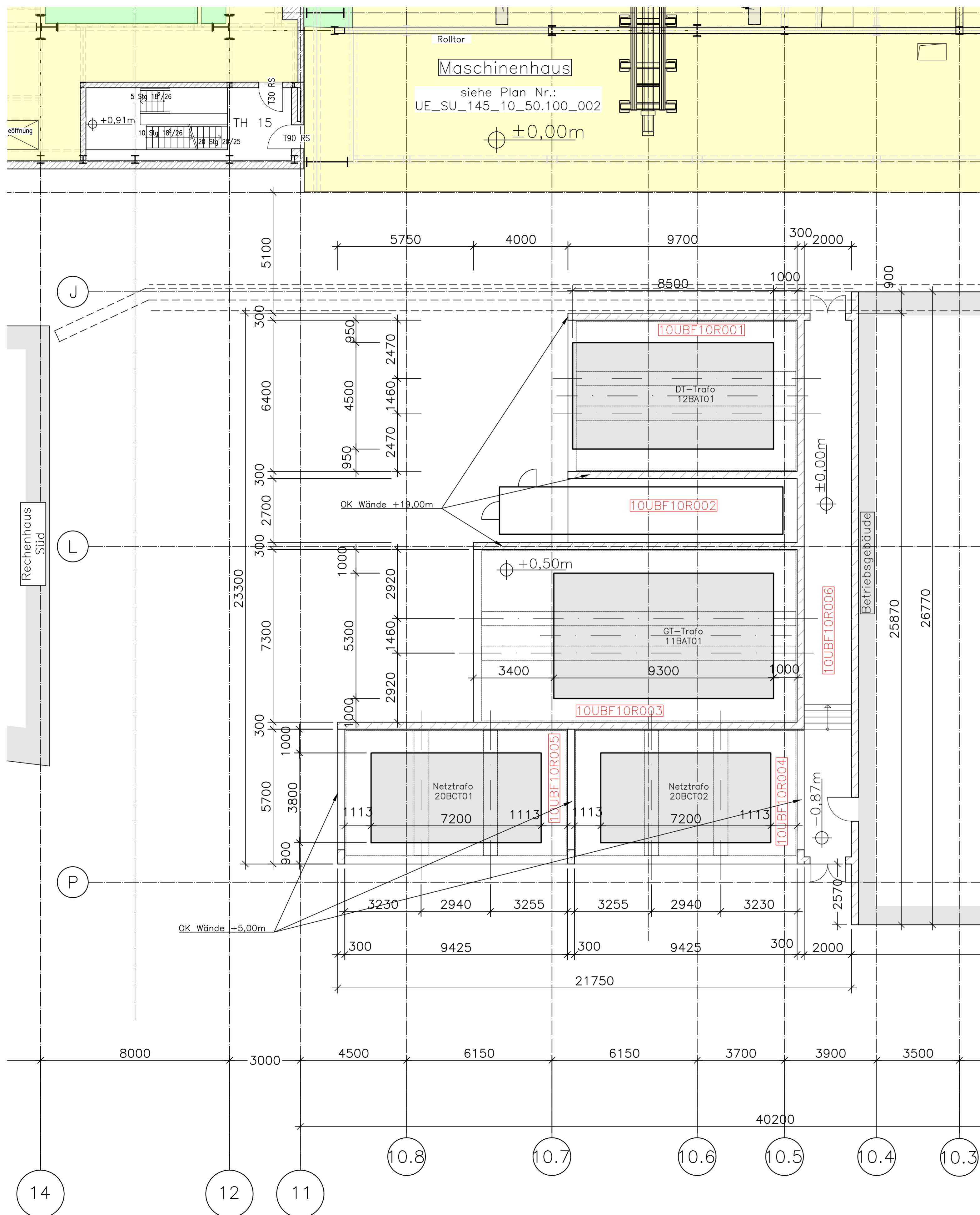
Grundriss ±0,00 (Trafos) M 1:100
