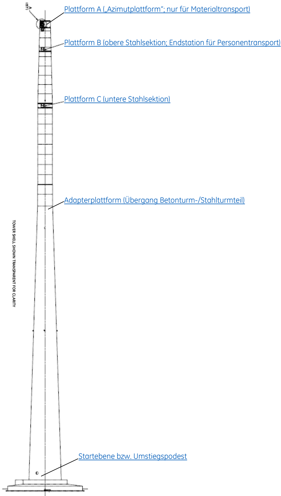
Abbildung 1. Übersicht der Turmplattformen im Betonhybridturm
