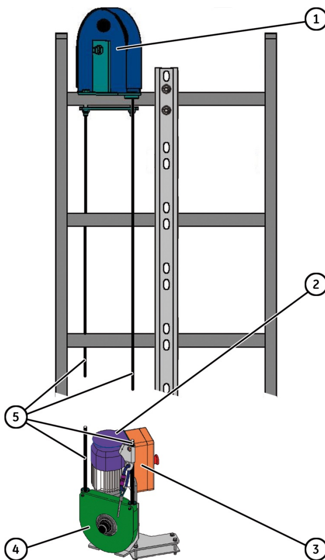
Abbildung 7: Beispiel einer Aufstiegshilfe
