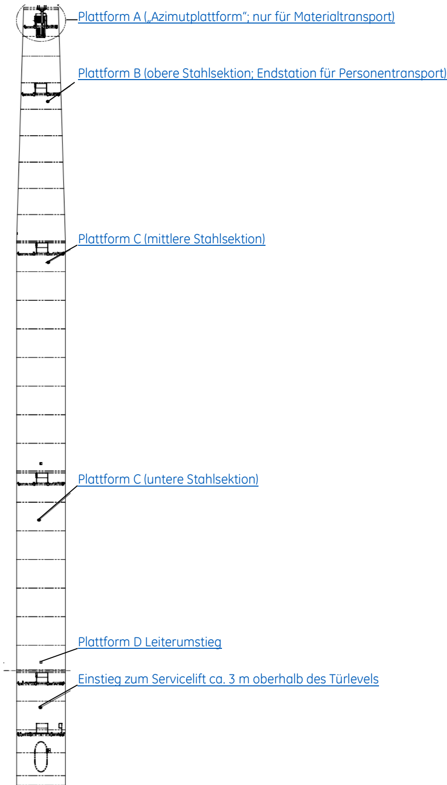
Abbildung 2: Übersicht der Turmplattformen im Stahlrohrturm
