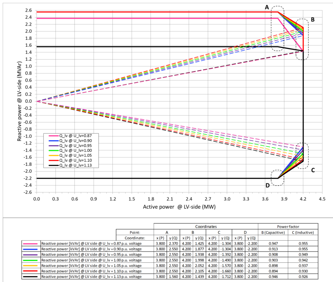
Abbildung 10-5: Blindleistungskapazität im leistungsoptimierten 4,2-MW-Modus (PO1)
