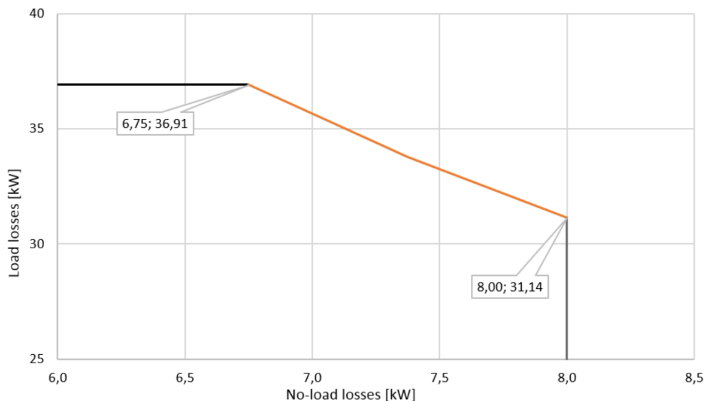
Abbildung 4-2 Transformatorverluste, zulässiger Bereich für Stufe 2
