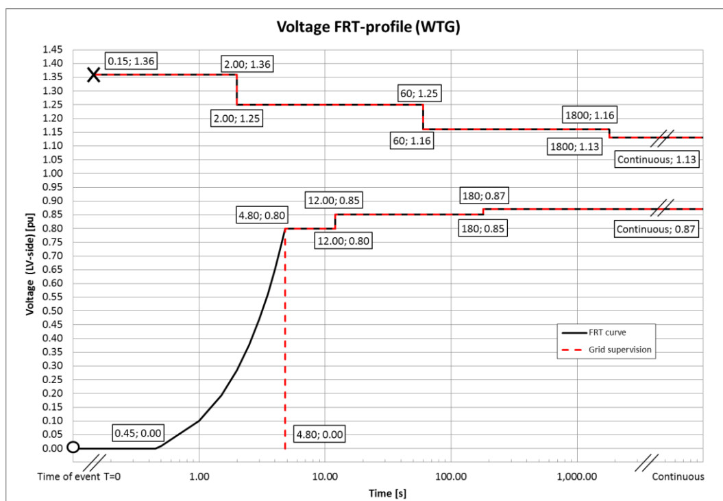
Abbildung 10-6: Spannungstoleranzkurve für symmetrische und asymmetrische Störungen, wobei U die gemessene Spannung im Stromnetz darstellt
