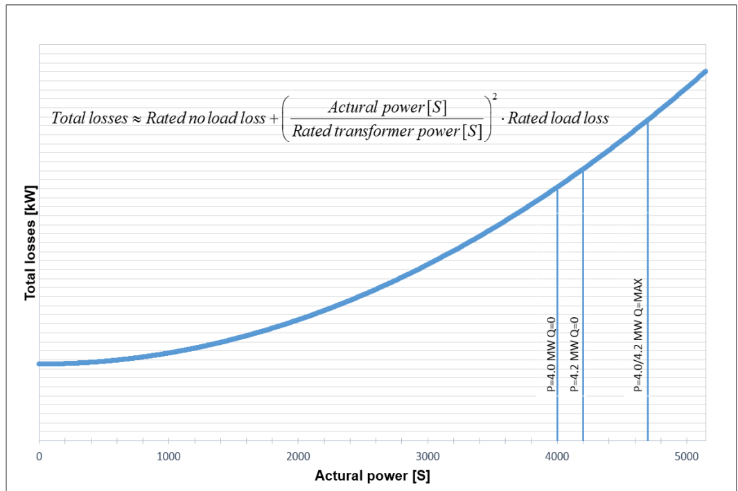
Abbildung 4-3: Gesamtverluste gegenüber Ist-Leistung.
