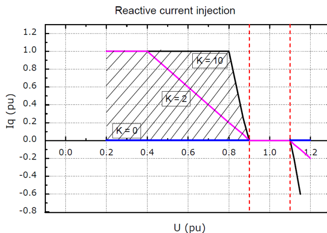
Abbildung 10-7: Blindstromeinspeisung
