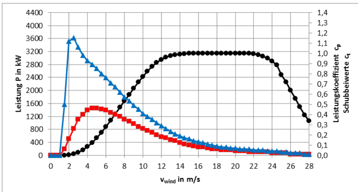
Abb. 3: Leistungs-, c_p - und c_t -Kennlinie E-138 EP3 E2 / 4200 kW Betriebsmodus 100,5 dB
