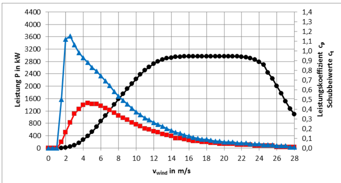
Abb. 4: Leistungs-, c_p - und c_t -Kennlinie E-138 EP3 E2 / 4200 kW Betriebsmodus 99,5 dB
