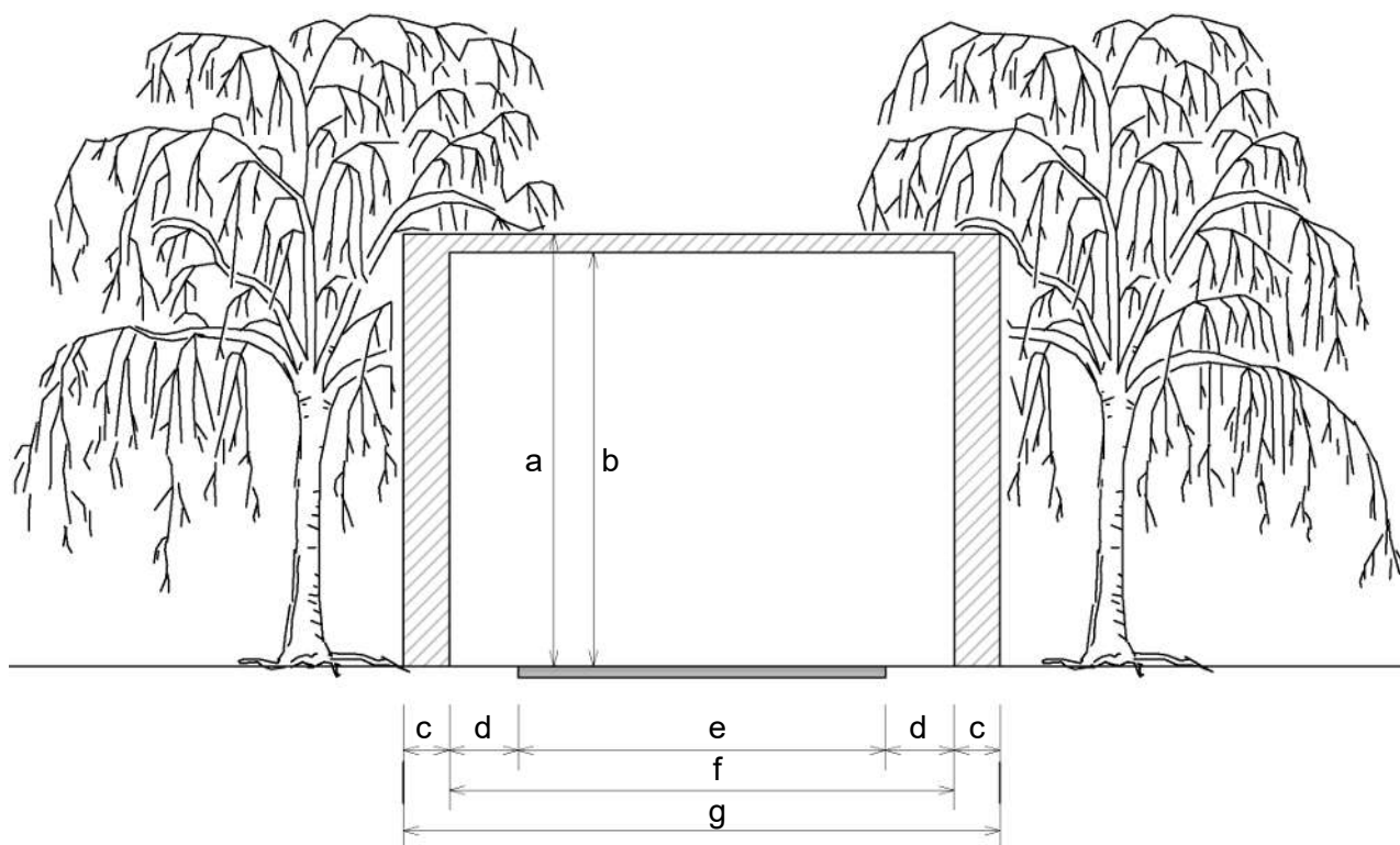
Abb. 5: Lichtraumprofil
