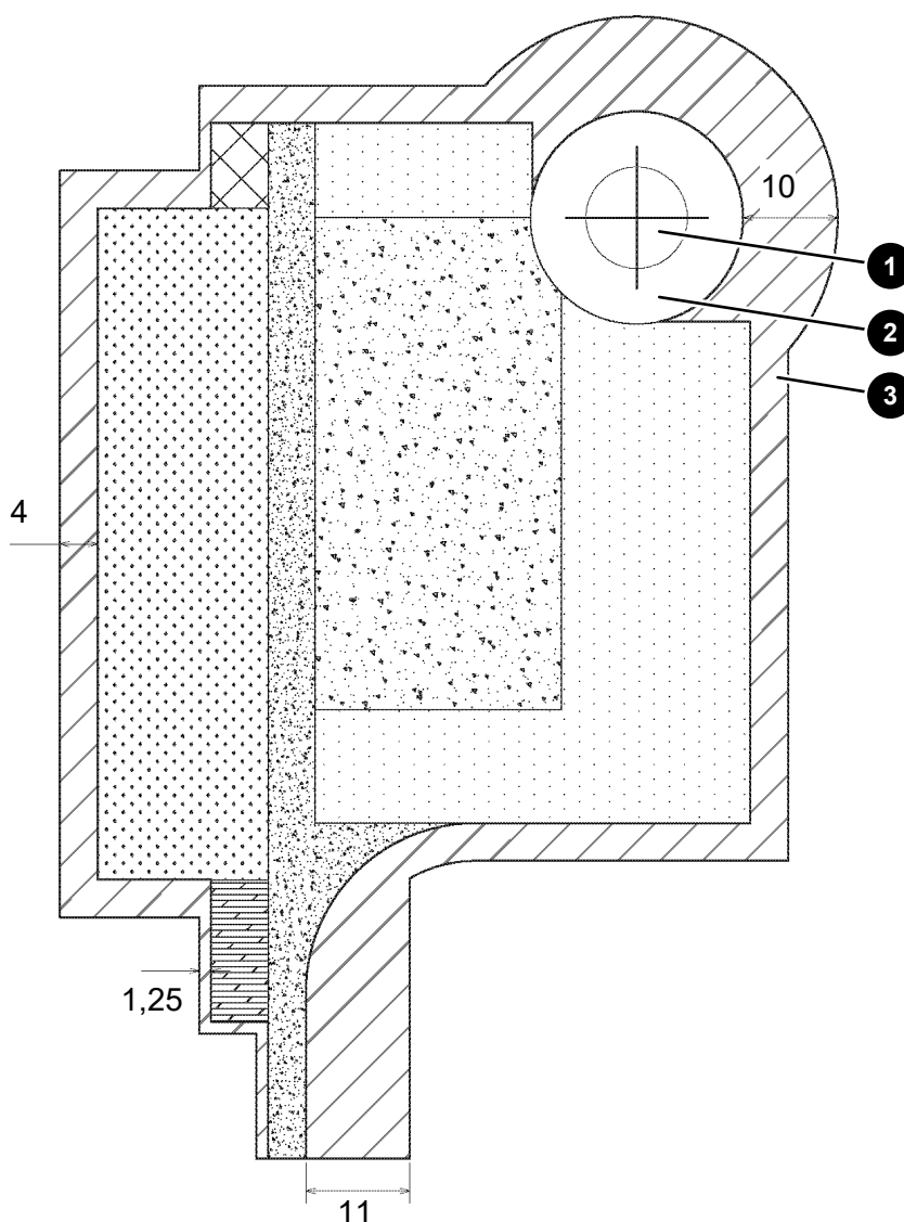
Abb. 8: Arbeitsbereich am WEA-Standort in Waldgebieten, Baumaß (alle Maßangaben in Meter)
