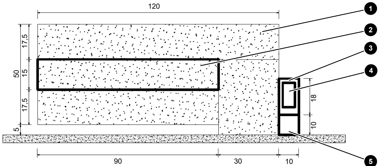
Abb. 10: Standard Logistikfläche, Baumaße und Zonen
