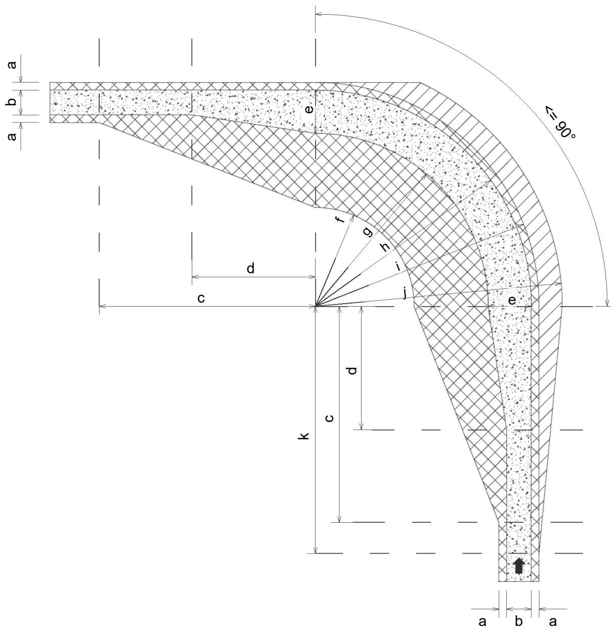
Abb. 2: 90-Grad-Kurve (Konstruktionsschema)
