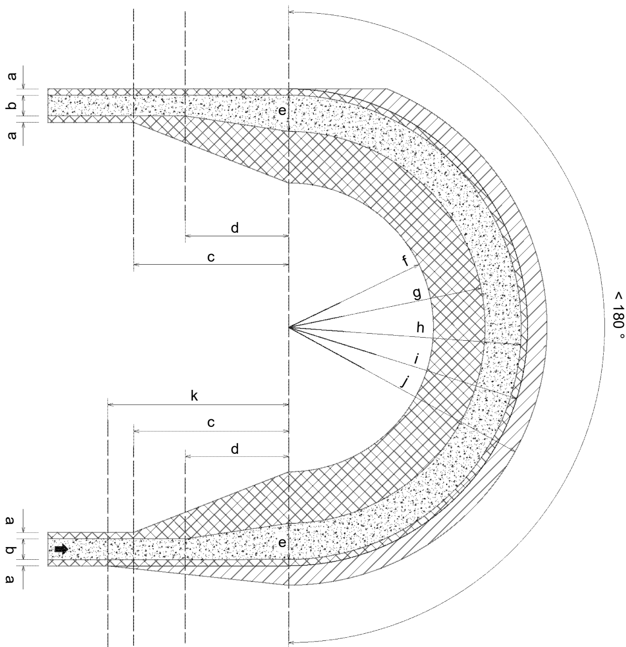
Abb. 3: 180-Grad-Kurve (Konstruktionsschema)
