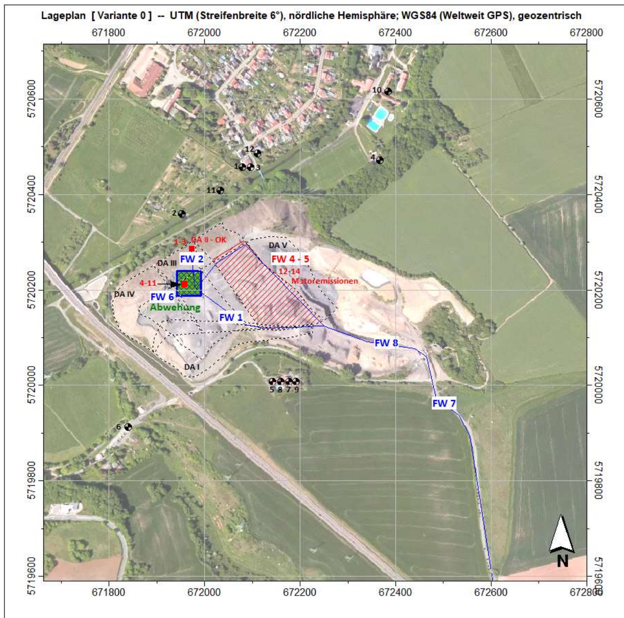
Abbildung 8.3: Verortung der Emissionsquellen Variante 3 / Beurteilungspunkte (BUP)
