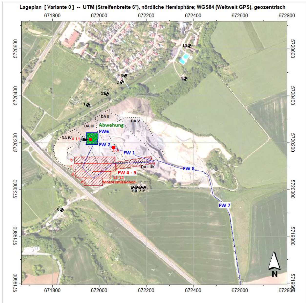
Abbildung 8.1: Verortung der Emissionsquellen Variante 1 / Beurteilungspunkte (BUP)
