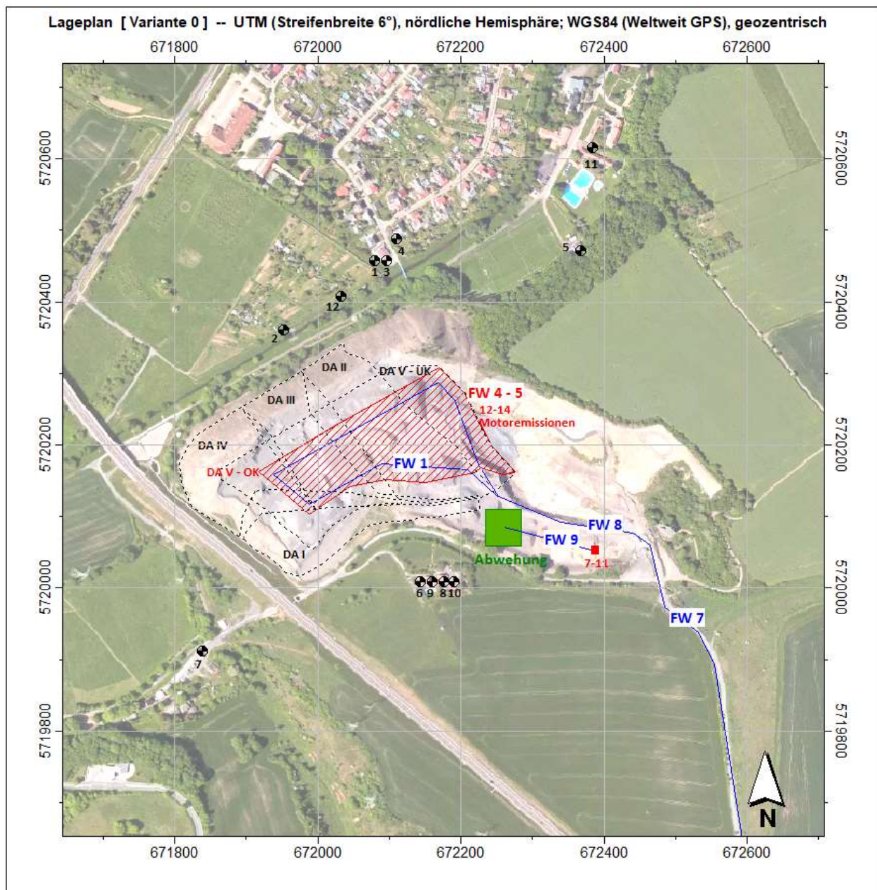
Abbildung 8.4: Verortung der Emissionsquellen Variante 4 / Beurteilungspunkte (BUP)
