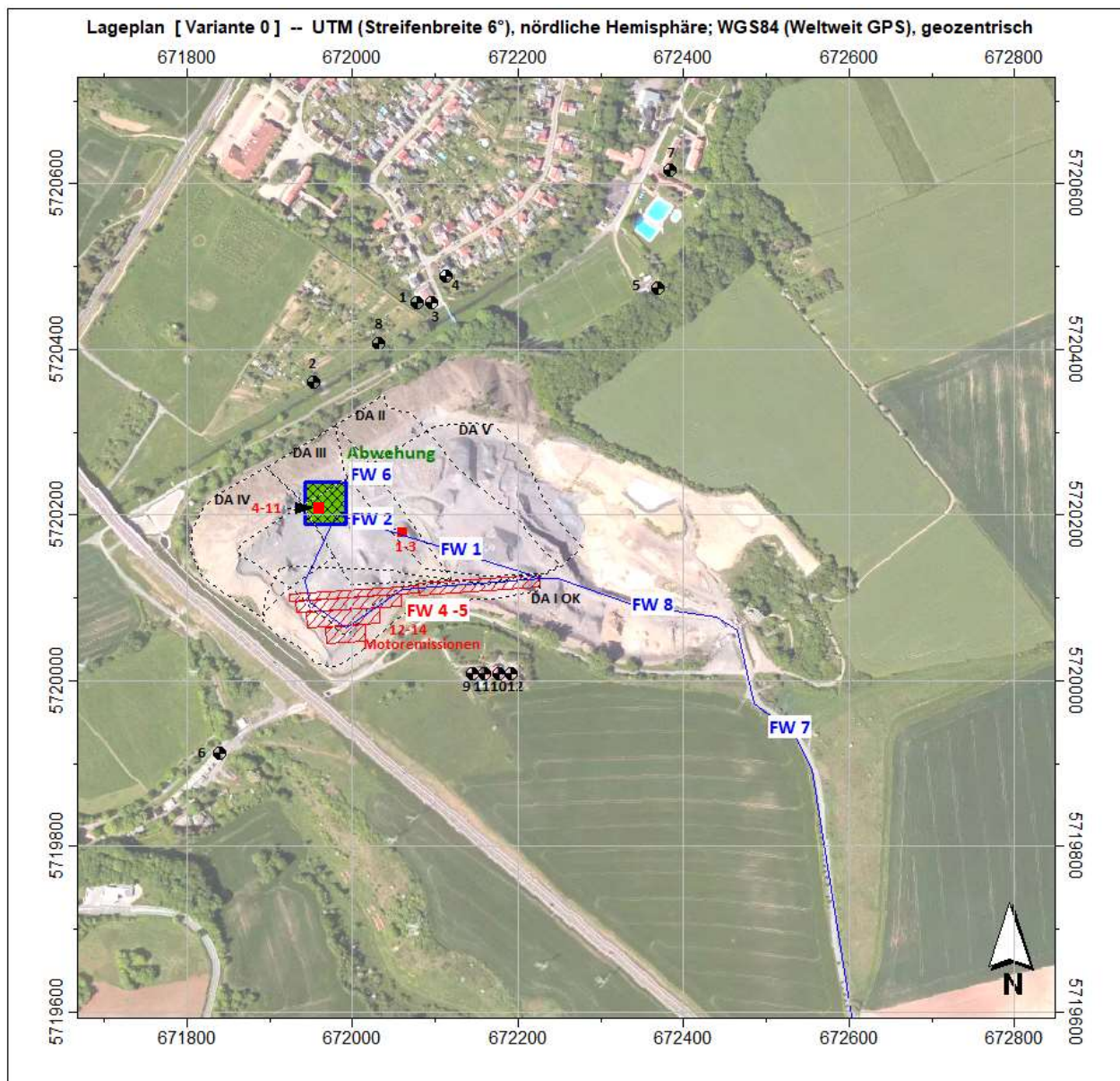
Abbildung 8.2: Verortung der Emissionsquellen Variante 2 / Beurteilungspunkte (BUP)
