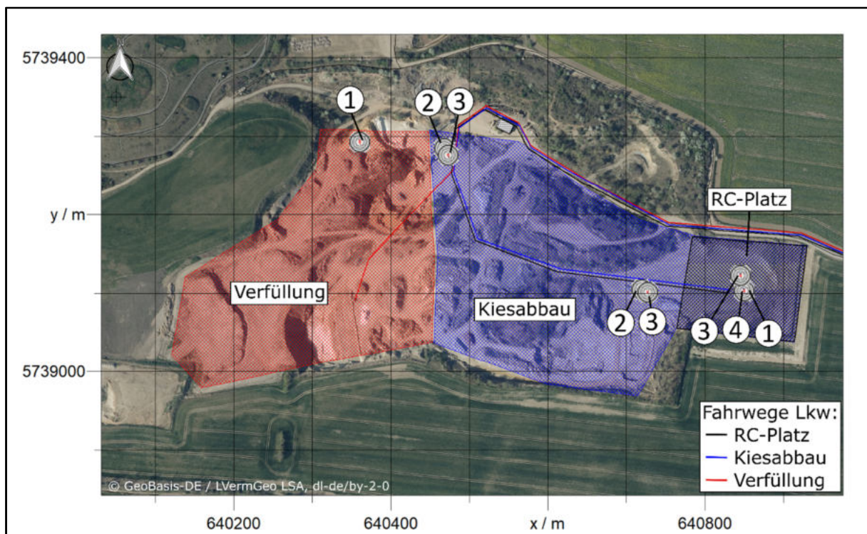
Abbildung 2: Schallquellen Szenario 1
