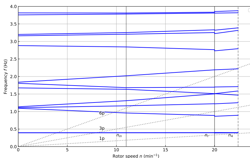
Abbildung A.2: Campbell-Diagramm des Simulationsmodells
