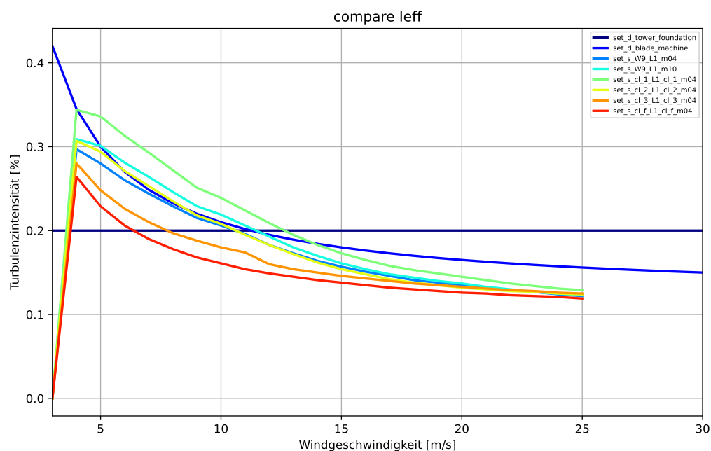
Abbildung 3.2: Effektive Turbulenzintensitäten
