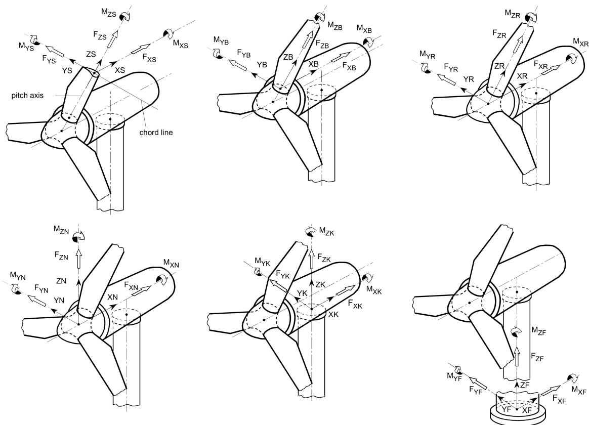
Abbildung 2.2: Verwendete Koordinatensysteme, nach [3]
