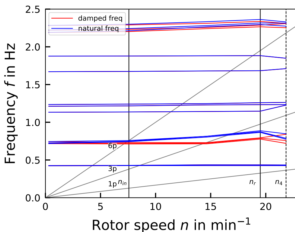
Abbildung A.2: Campbell-Diagramm des Simulationsmodells
