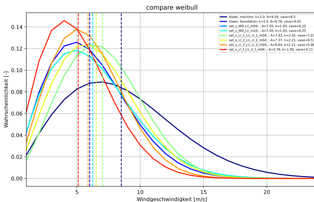
Abbildung 3.1: Vergleich der Weibull-Verteilungen
