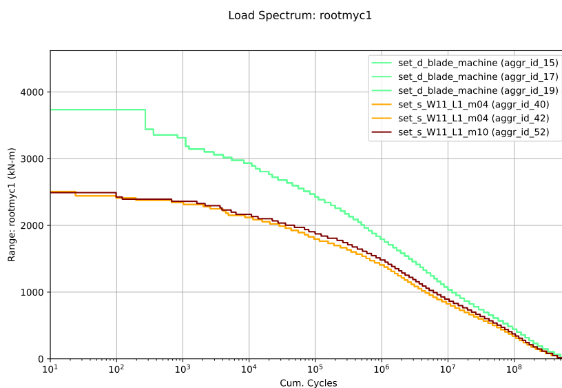
Abbildung B.8: Lasten am Rotorblatt ( M_{YS} ) im Bereich der Blattwurzel
