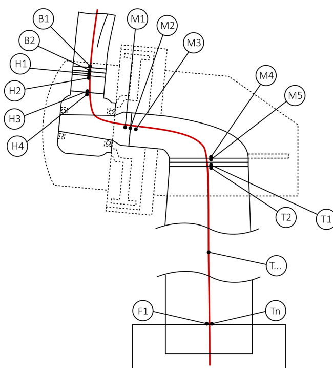
Abbildung 2.1: Betrachtete Komponenten im Hauptlastpfad (rot)
