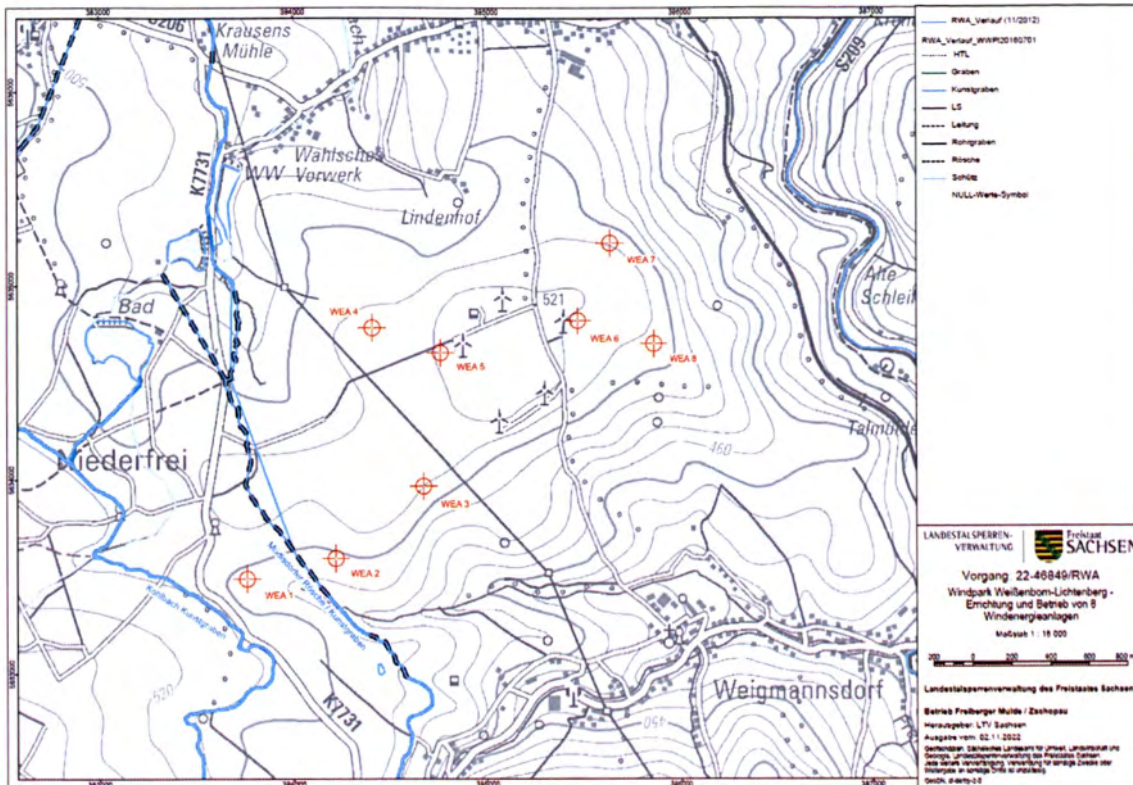
Abb 1.: Übersichtsplan
