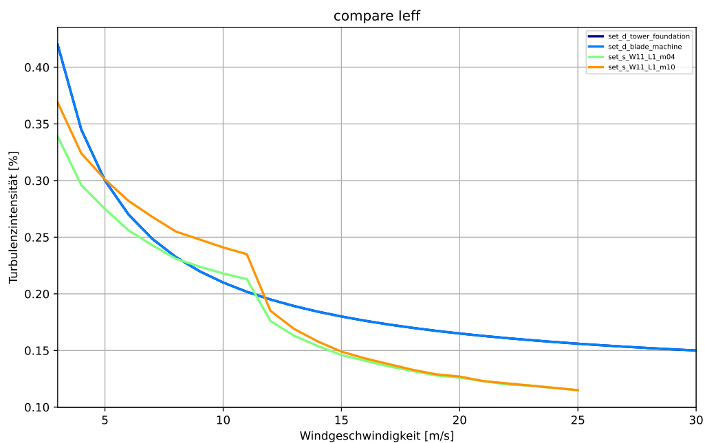
Abbildung 3.2: Effektive Turbulenzintensitäten
