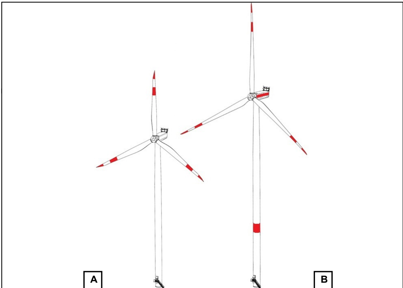
Abb. 1: Übersicht Kennzeichnungsmerkmale bei Anlagen 100 - 150 m (A) und >150 m (B) in Deutschland bei Tag
