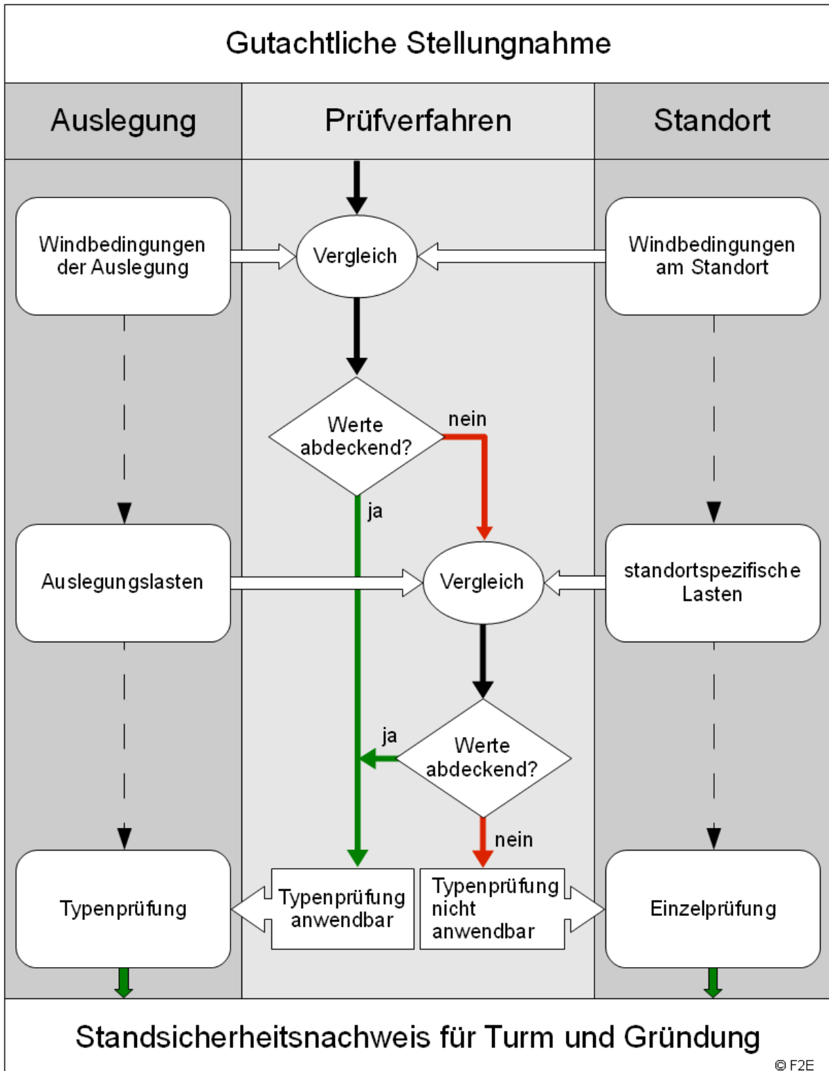
Abbildung 2.1.1: Schematische Darstellung des Prüfoerfahrens.
