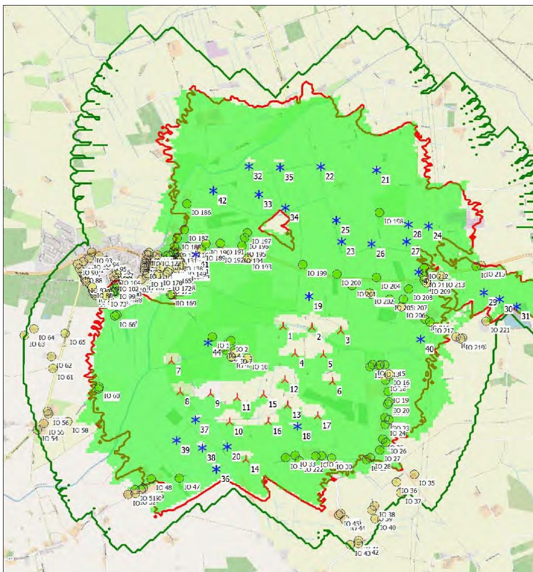
Abb. 4.1.4: Isolinien der Schattenwurfbelastung nach Umsetzung aller Planungen (Akustik Busch GmbH)
