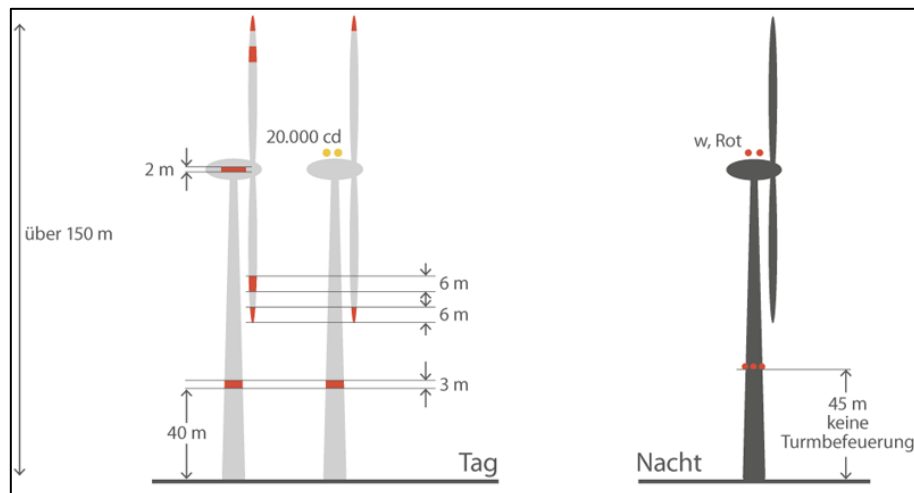
Abb. 1.3.1: Kennzeichnung von &gt; 150m-WEA (Prinzipskizze)
