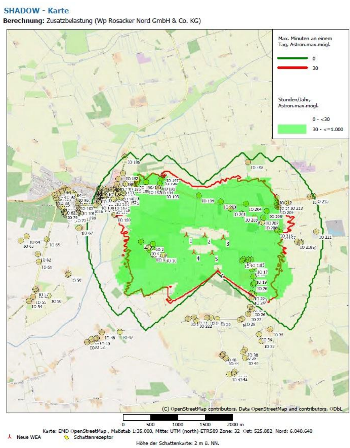
Abb. 4.1.5: Zusatzbelastung durch den WP Rosacker Nord (Akustik Busch 2024b)
