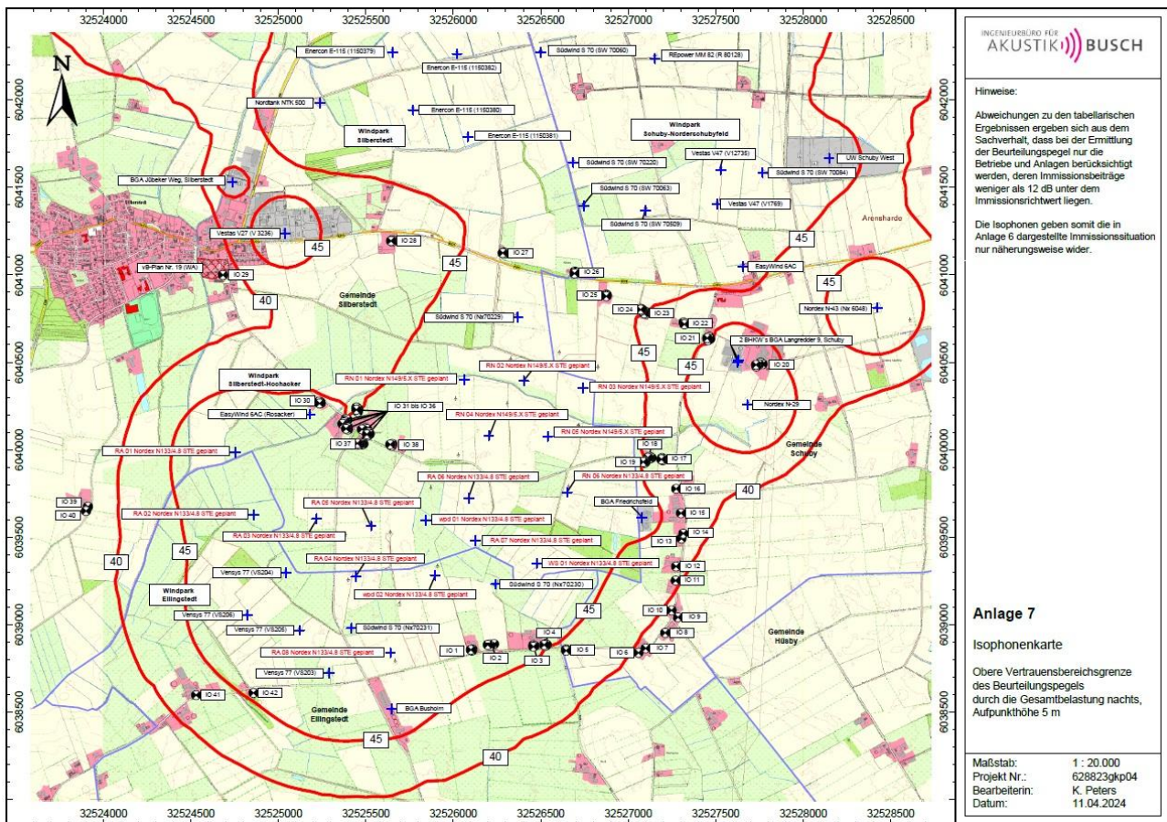
Abb. 4.1.3: Gesamtbelastung – nächtliche Immissionswerte - aus dem Schallgutachten (Akustik Busch GmbH, April 2024)
