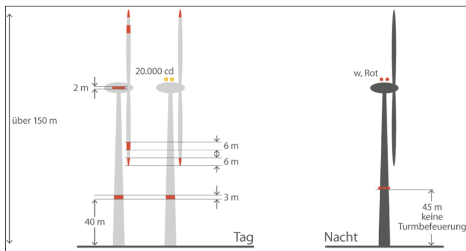
Abb. 3.1.1: Kennzeichnung von > 150m-WEA (Prinzipiskizze)
