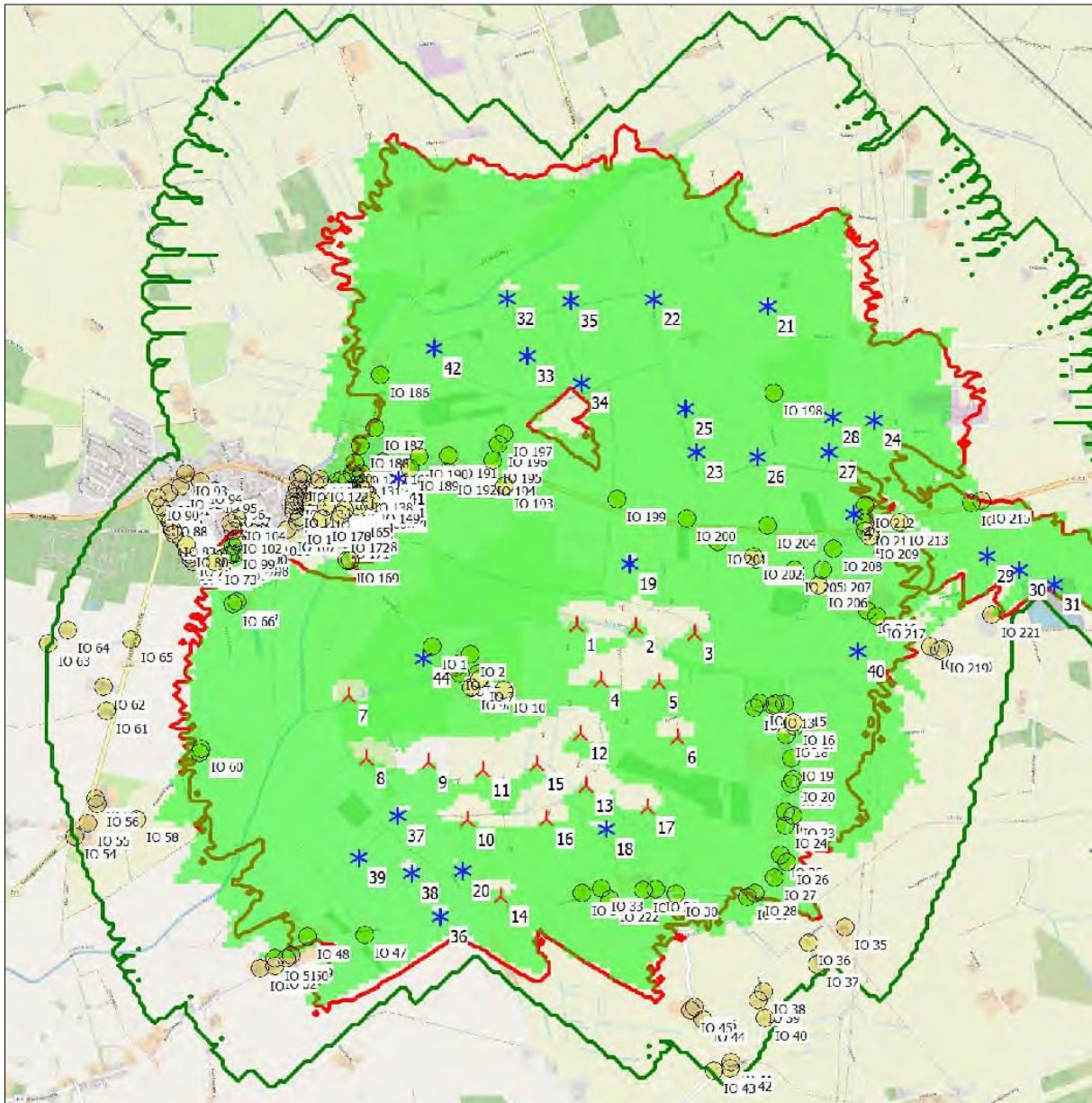
Abb. 4.1.7: Isolinen der Schattenwurfbelastung nach Umsetzung aller Planungen (Akustik Busch GmbH)
