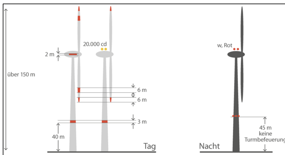
Abb. 1.3.1: Kennzeichnung von > 150m-WEA (Prinzipiskizze)
