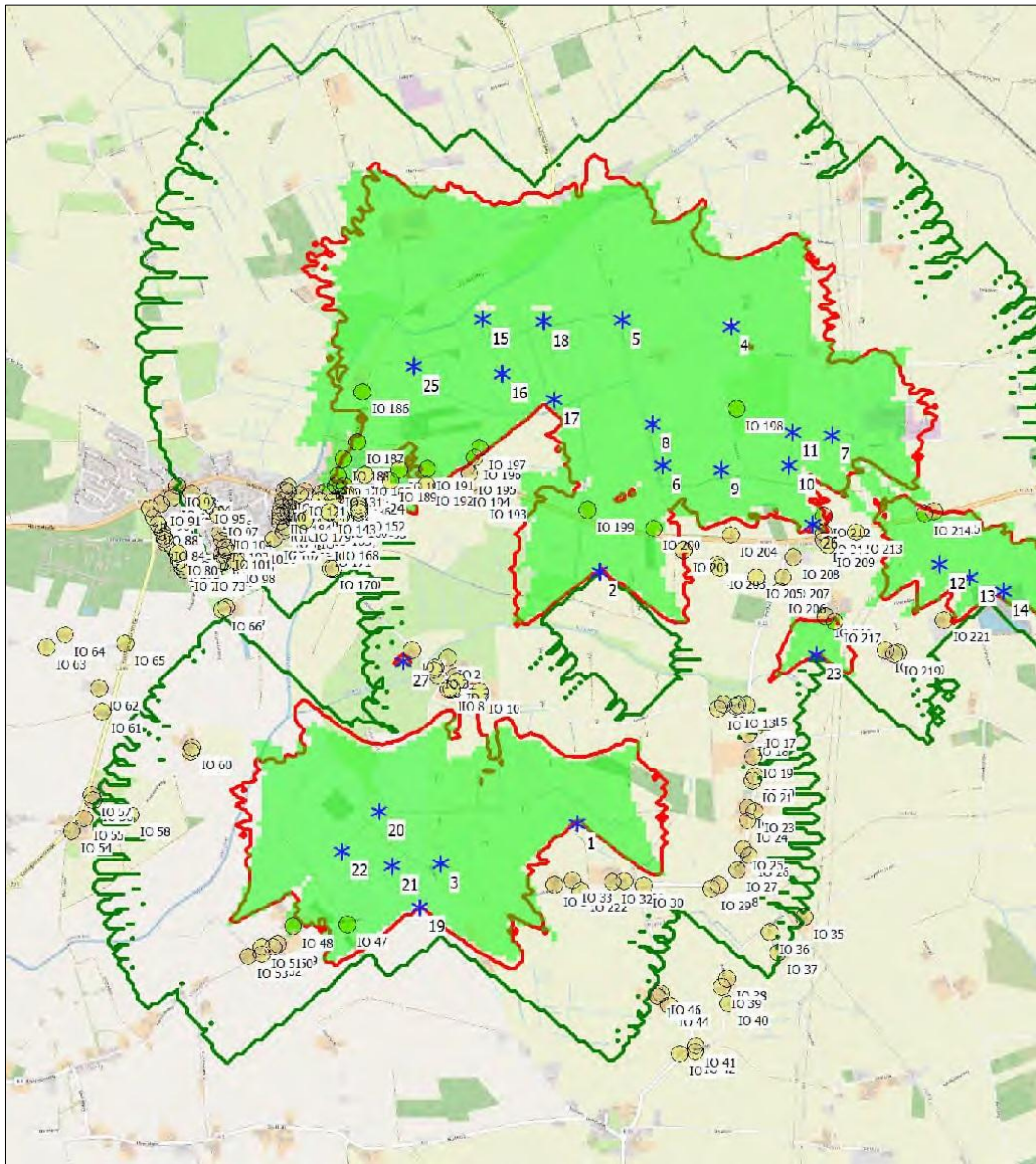
Abb. 4.1.3: Lage der Immissionsorte und Vorbelastung - ohne die abzubauenen Altanlagen (Akustik Busch GmbH)
