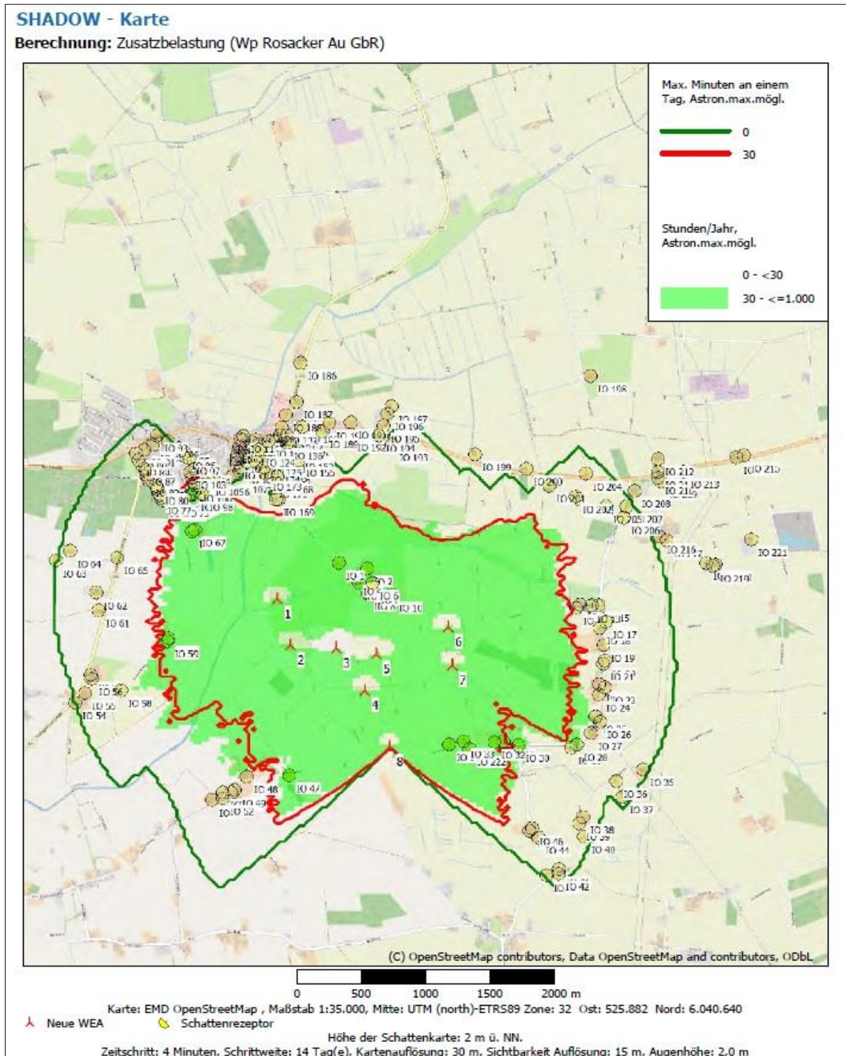
Abb. 4.1.6: Zusatzbelastung durch den WP Rosacker Au (Akustik Busch 2024b)
