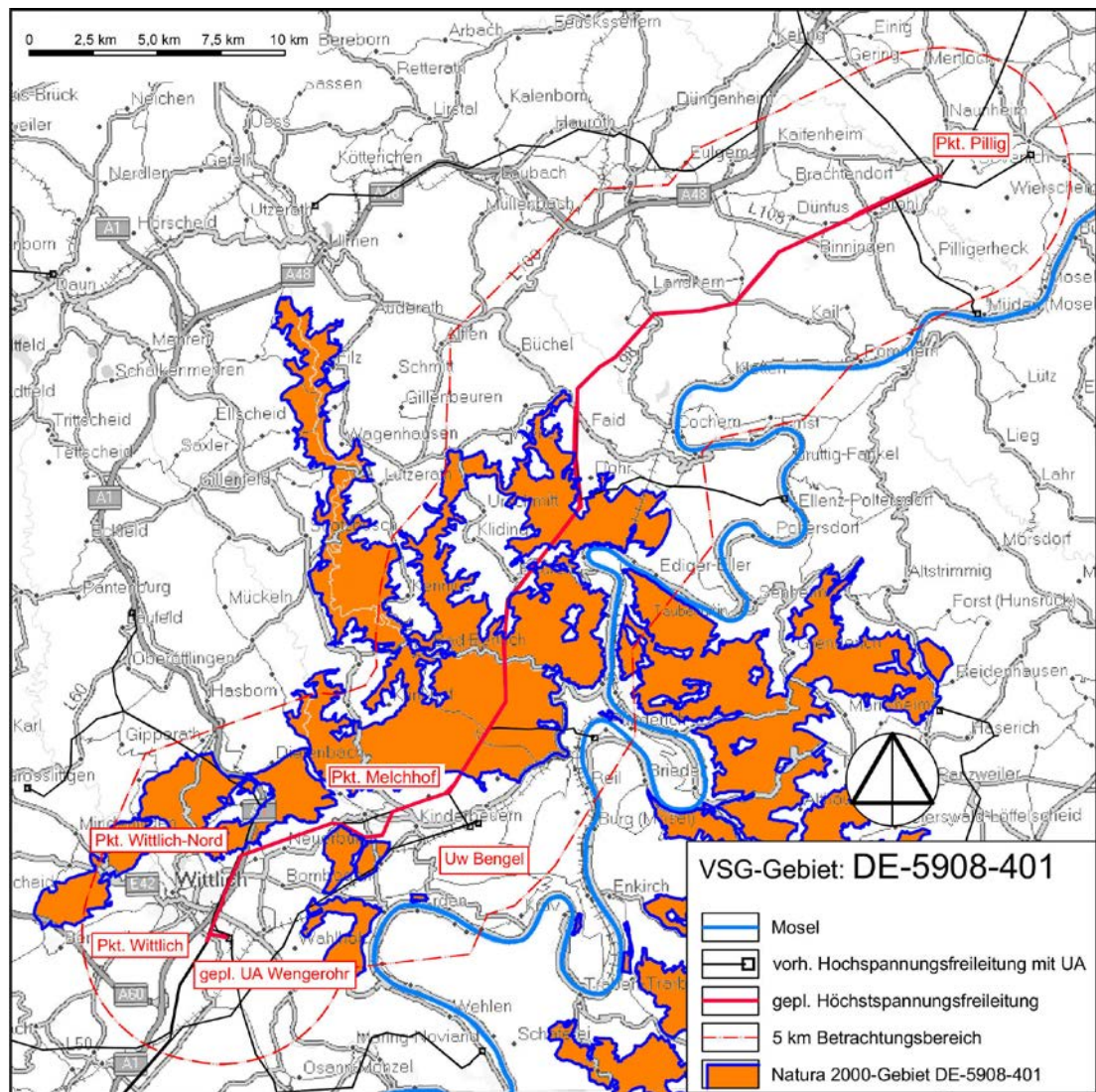
Abb. 1: Übersicht des Natura 2000-Gebietes "Wälder zwischen Wittlich und Cochem" (DE-5908-401)
