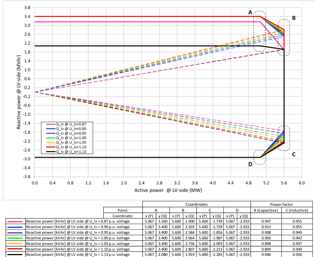
Abbildung 3-2: Blindleistungskapazität.
