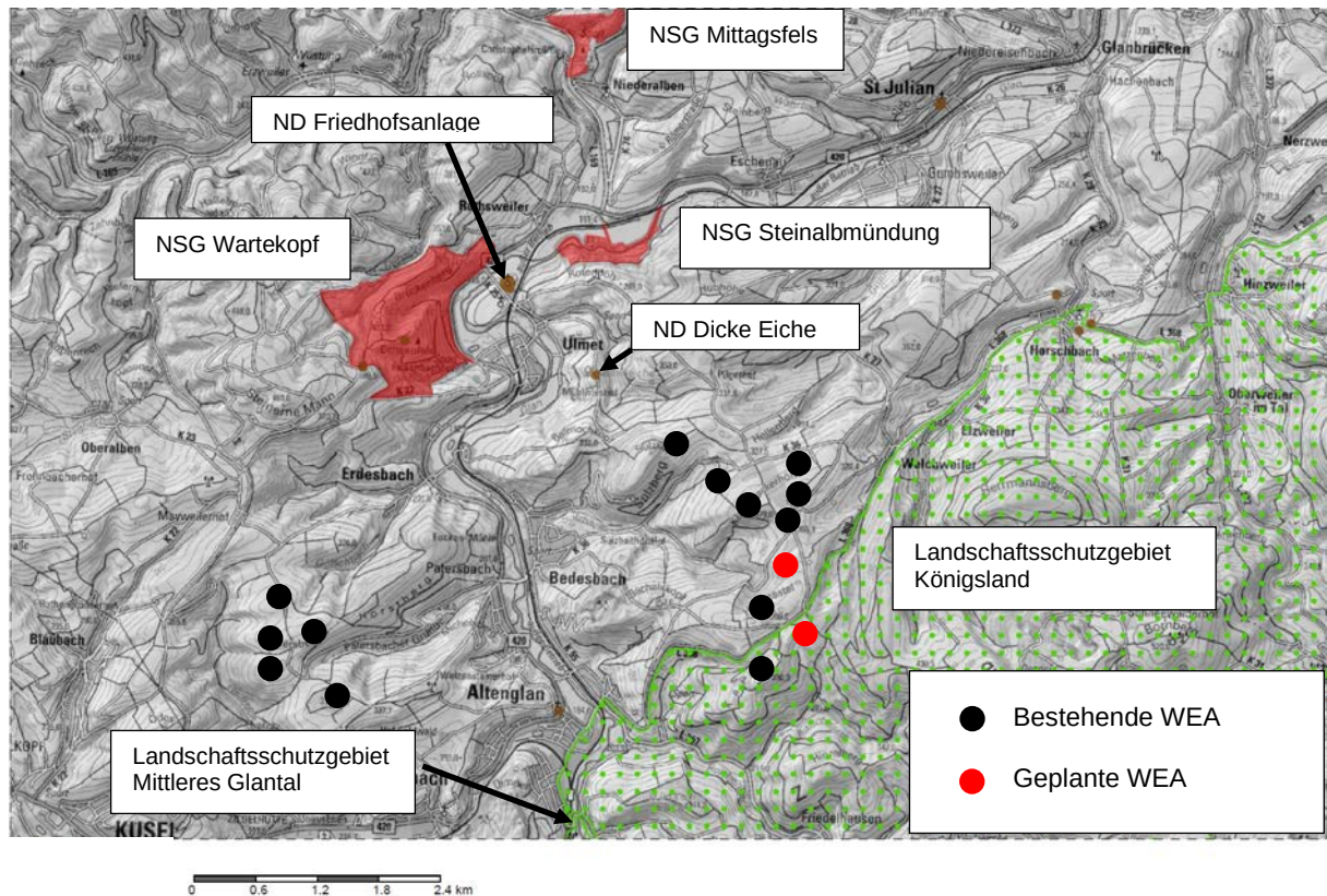
Abbildung 6: Übersicht über die Lage der sonstigen Schutzgebiete in der näheren und weiteren Umgebung der geplanten Windenergieanlagen
