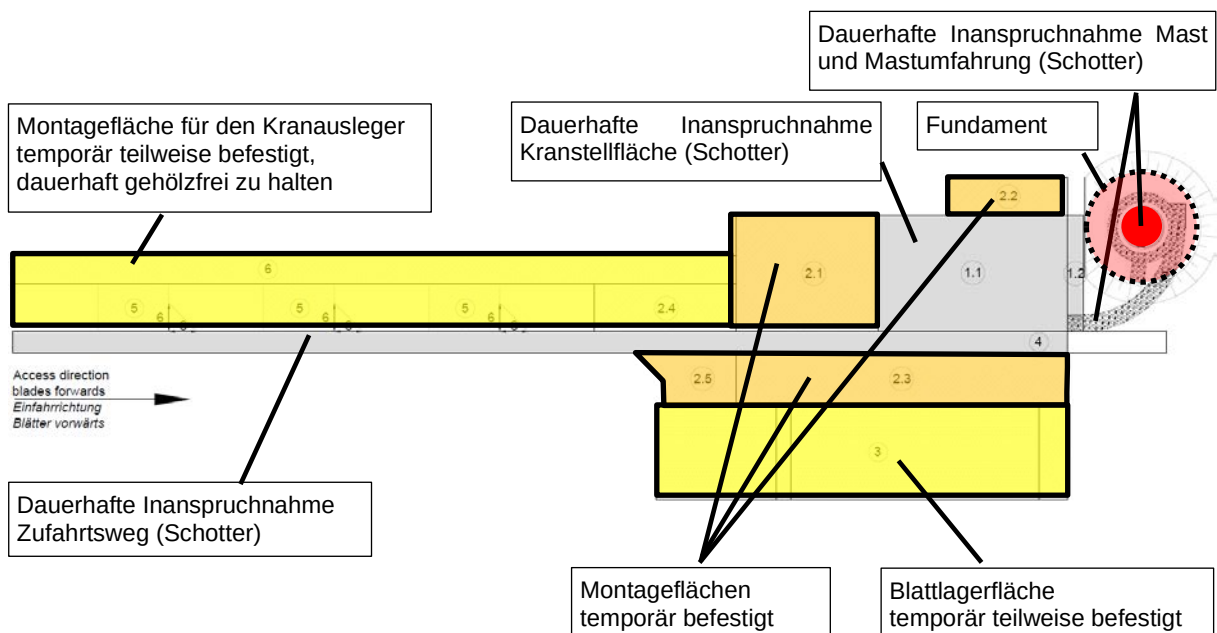
Abbildung 23: Systemskizze für Kranaufstellfläche, Turmfundament und Arbeitsbereiche
