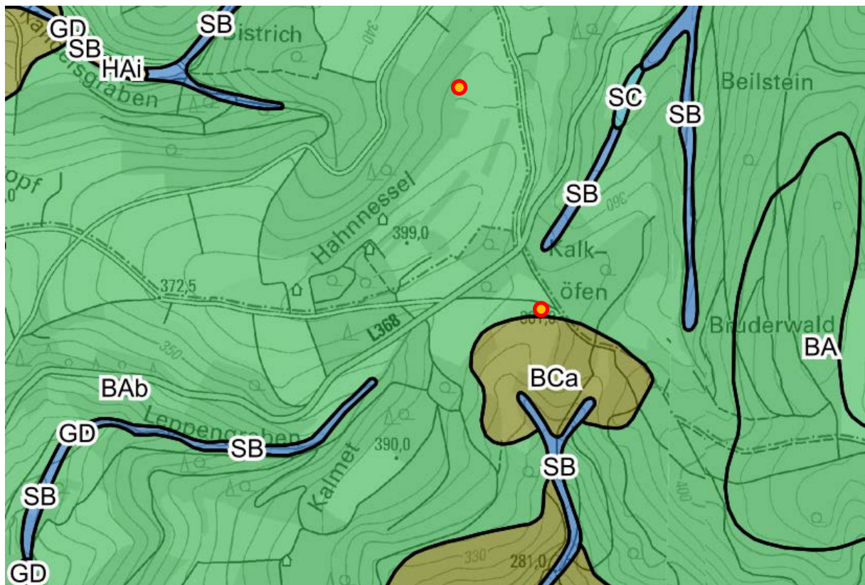
Abbildung 11: Heutige potenziell natürliche Vegetation
