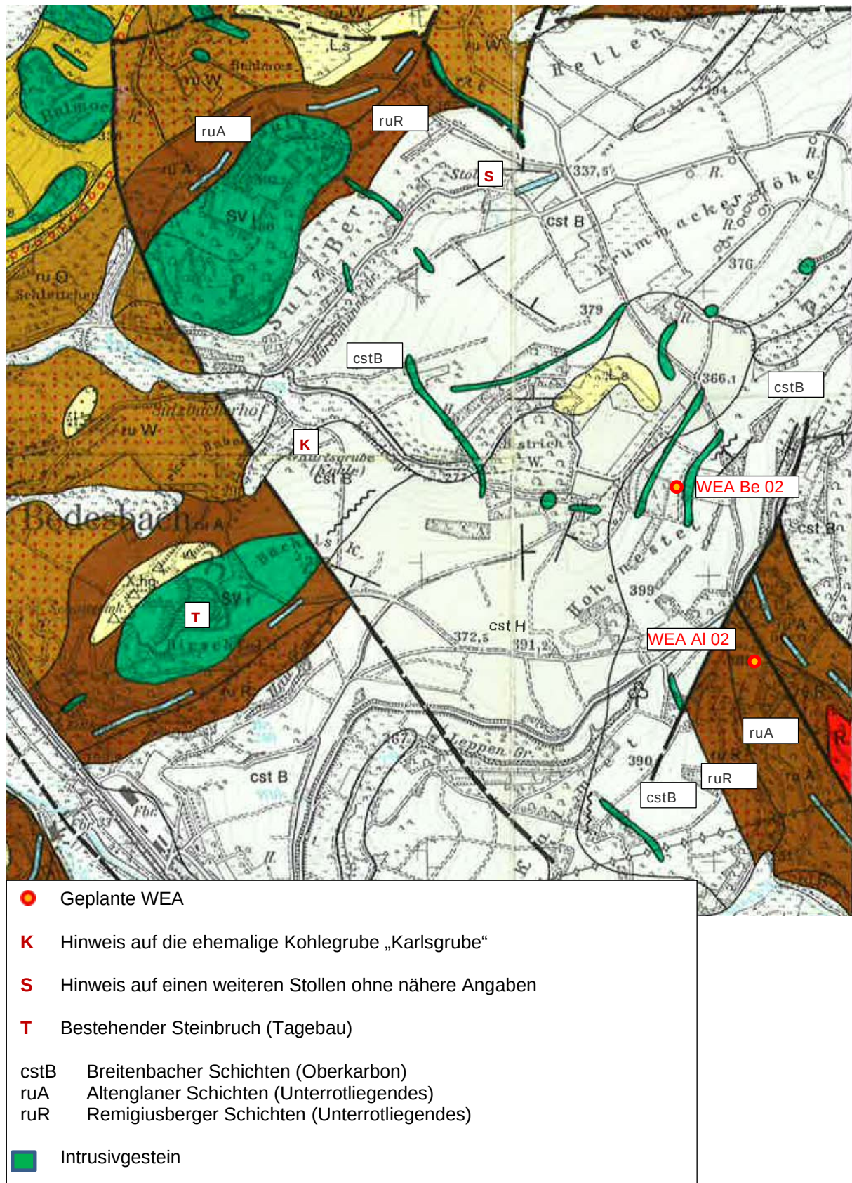
Abbildung 9: Auszug aus der geologischen Karte
