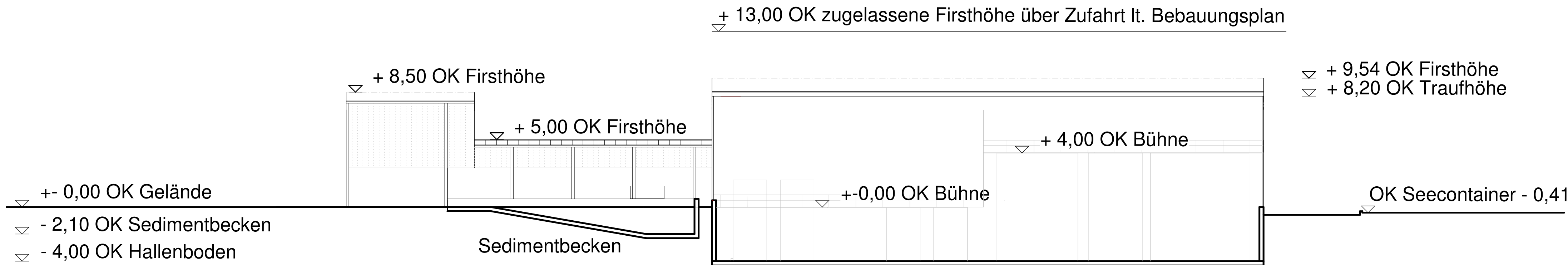
Längsschnitt
