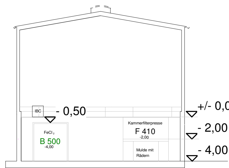
Schnitt C-C
