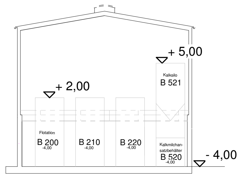
Schnitt A-A
