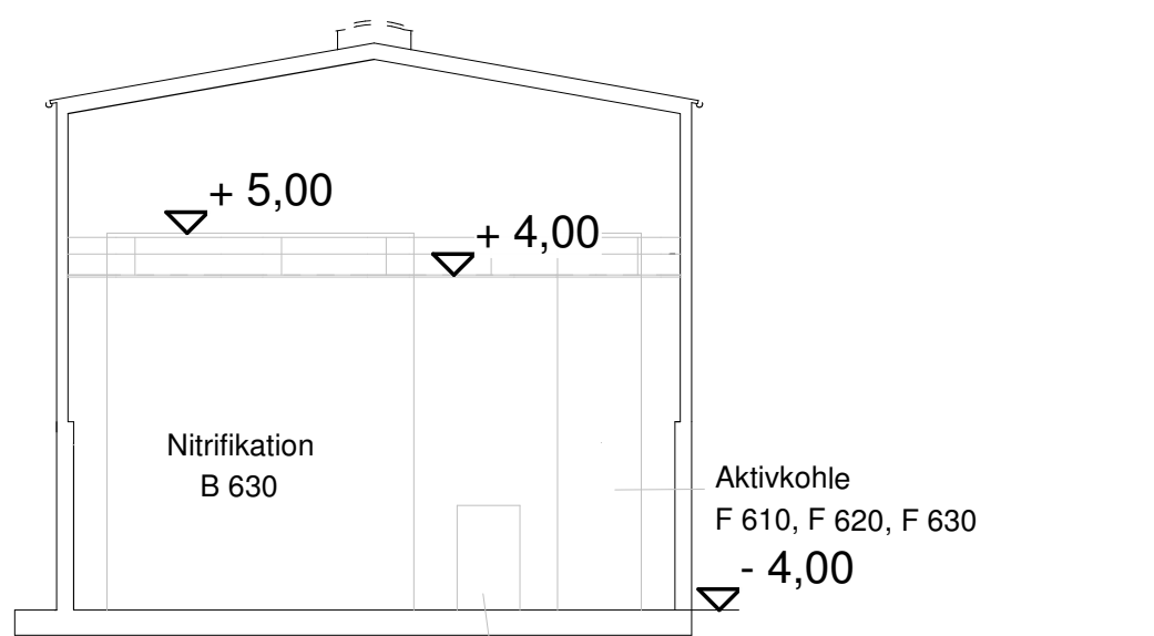
Schnitt F-F
