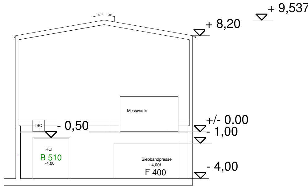
Schnitt D-D
