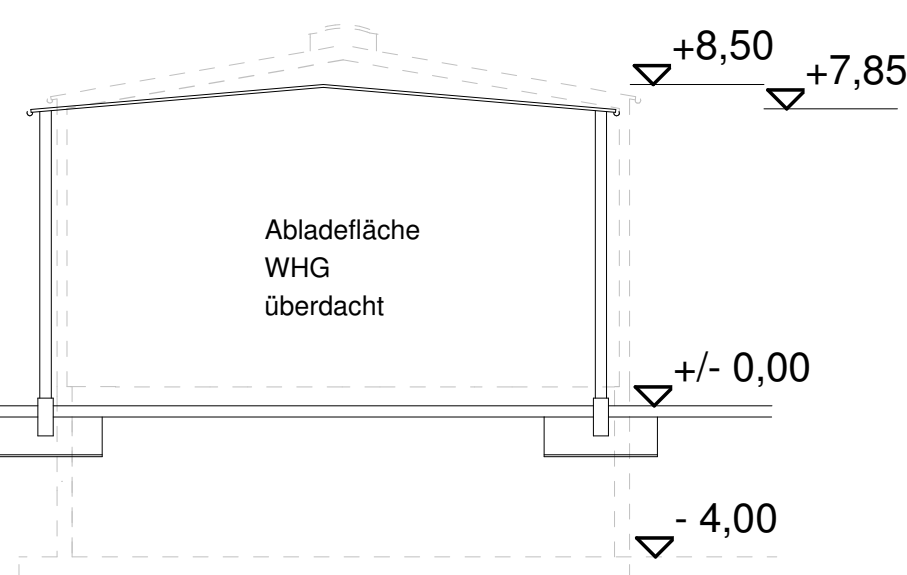
Schnitt G-G
