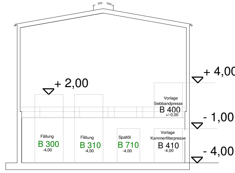
Schnitt B-B
