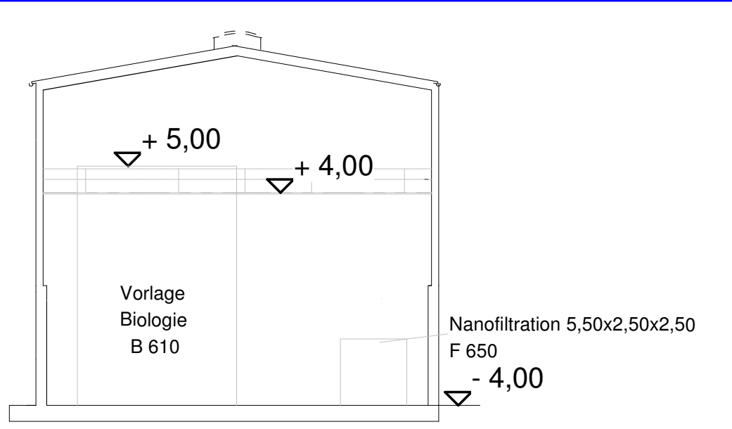
Schnitt E-E
