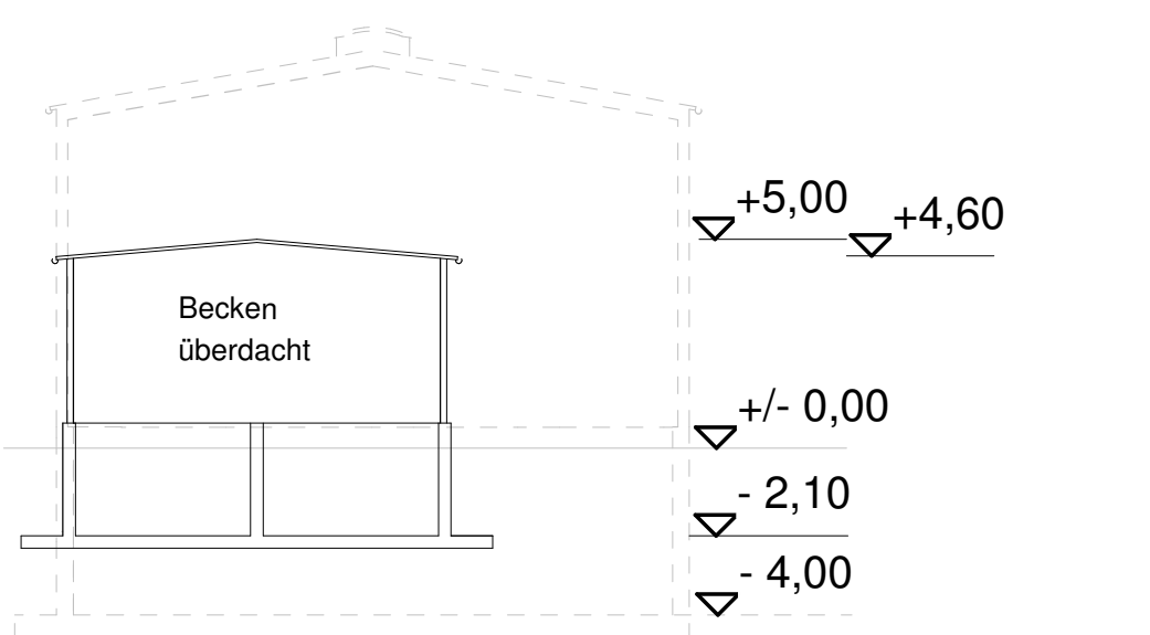
Schnitt H-H
