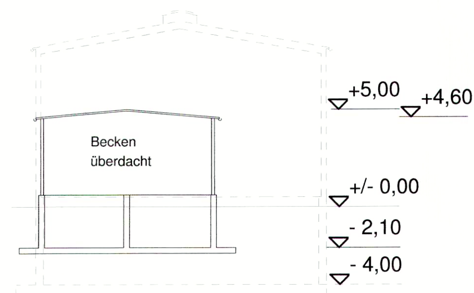
Schnitt H-H
