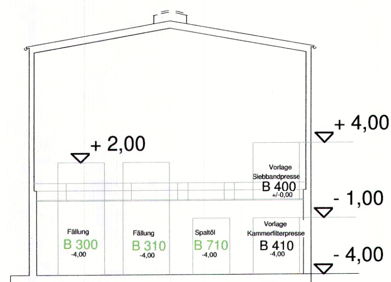
Schnitt B-B
