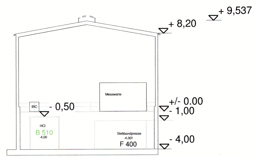
Schnitt D-D
