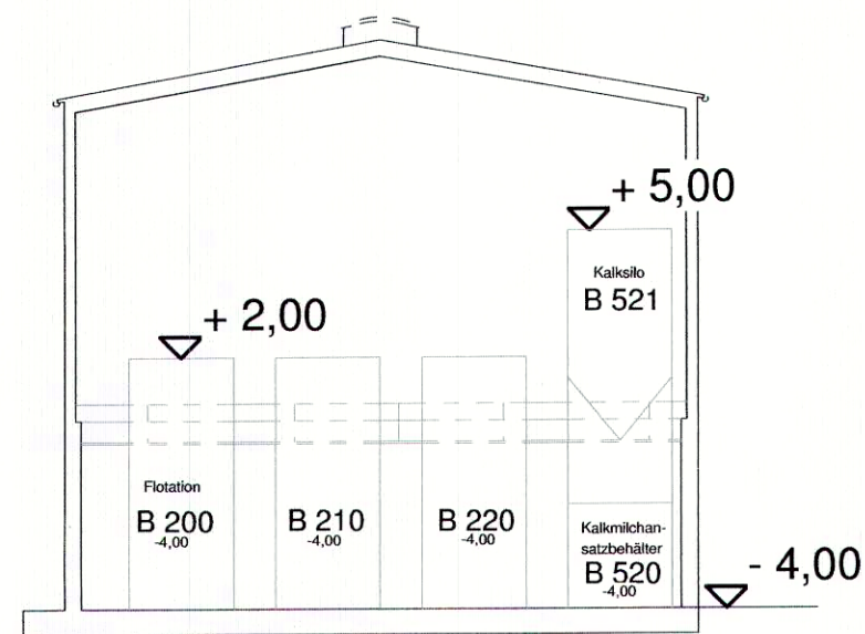
Schnitt A-A
