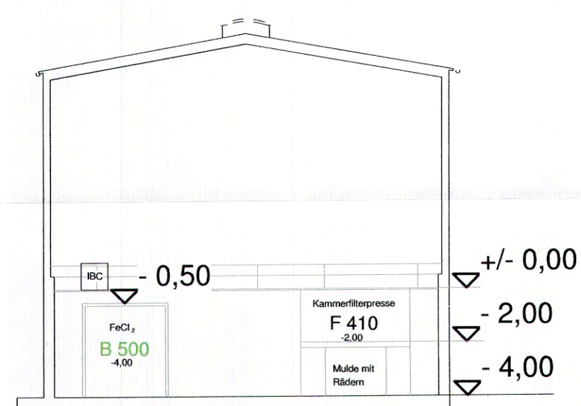
Schnitt C-C
