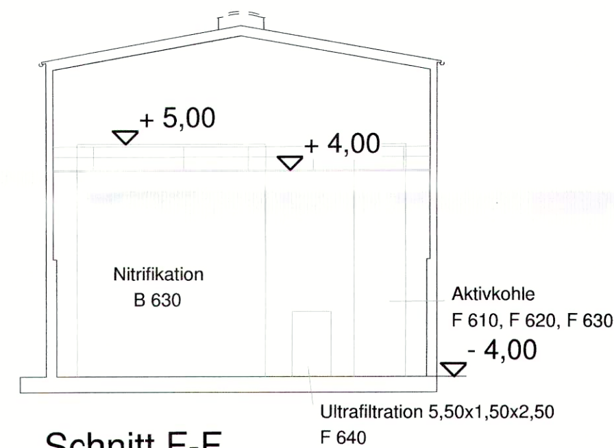
Schnitt F-F
