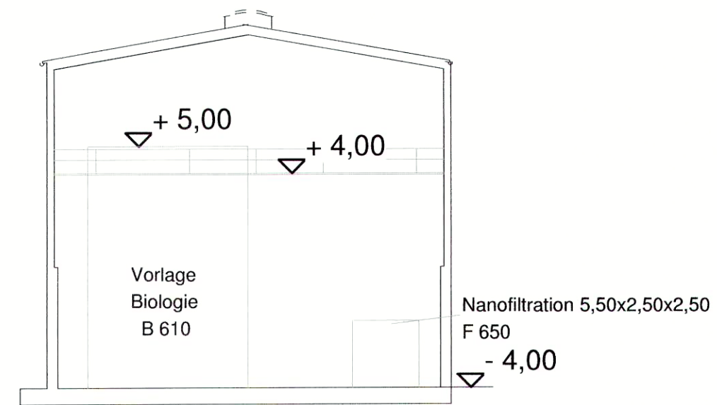
Schnitt E-E
