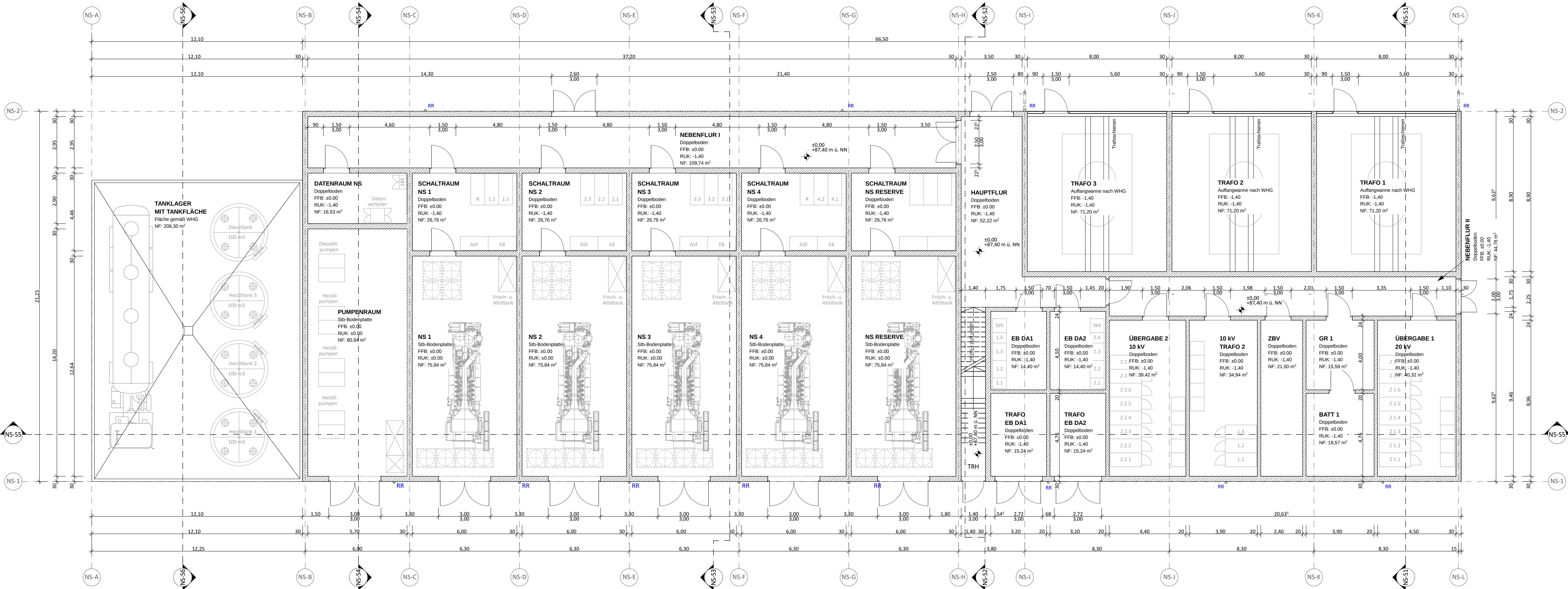
NEA-GEBÄUDE ERDGESCHOSS
