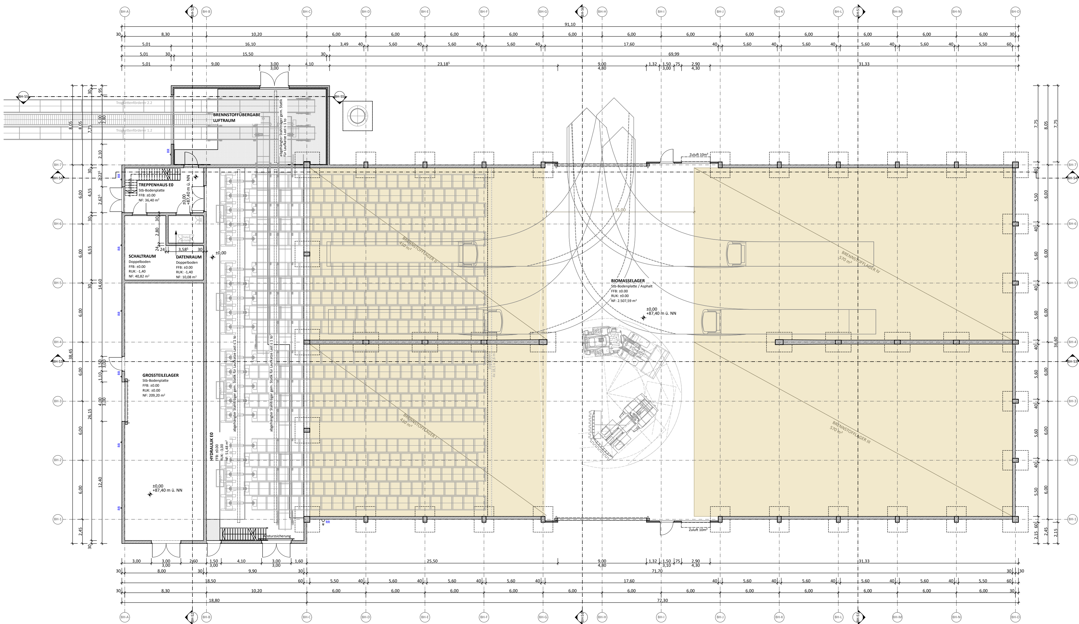
BRENNSTOFFLAGERHALLE ERDGESCHOSS
