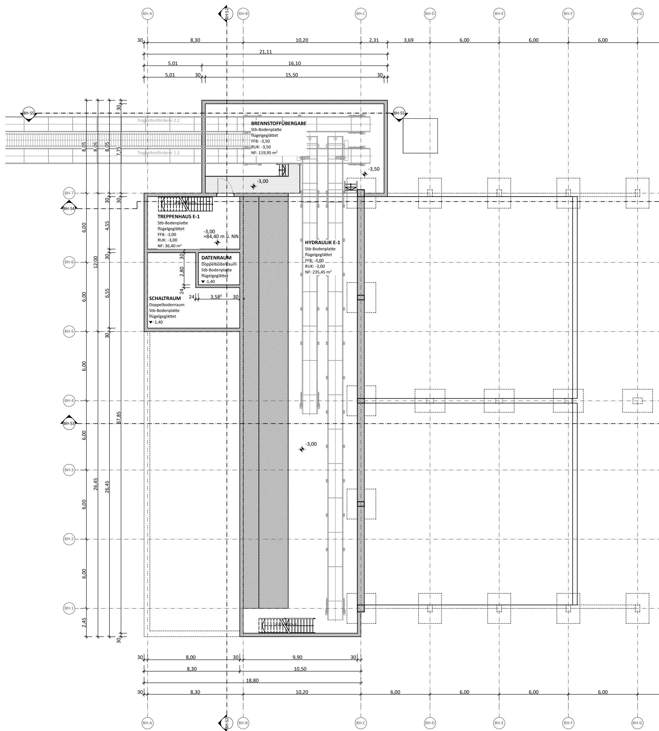
BRENNSTOFFLAGERHALLE KELLERGEOSCH
