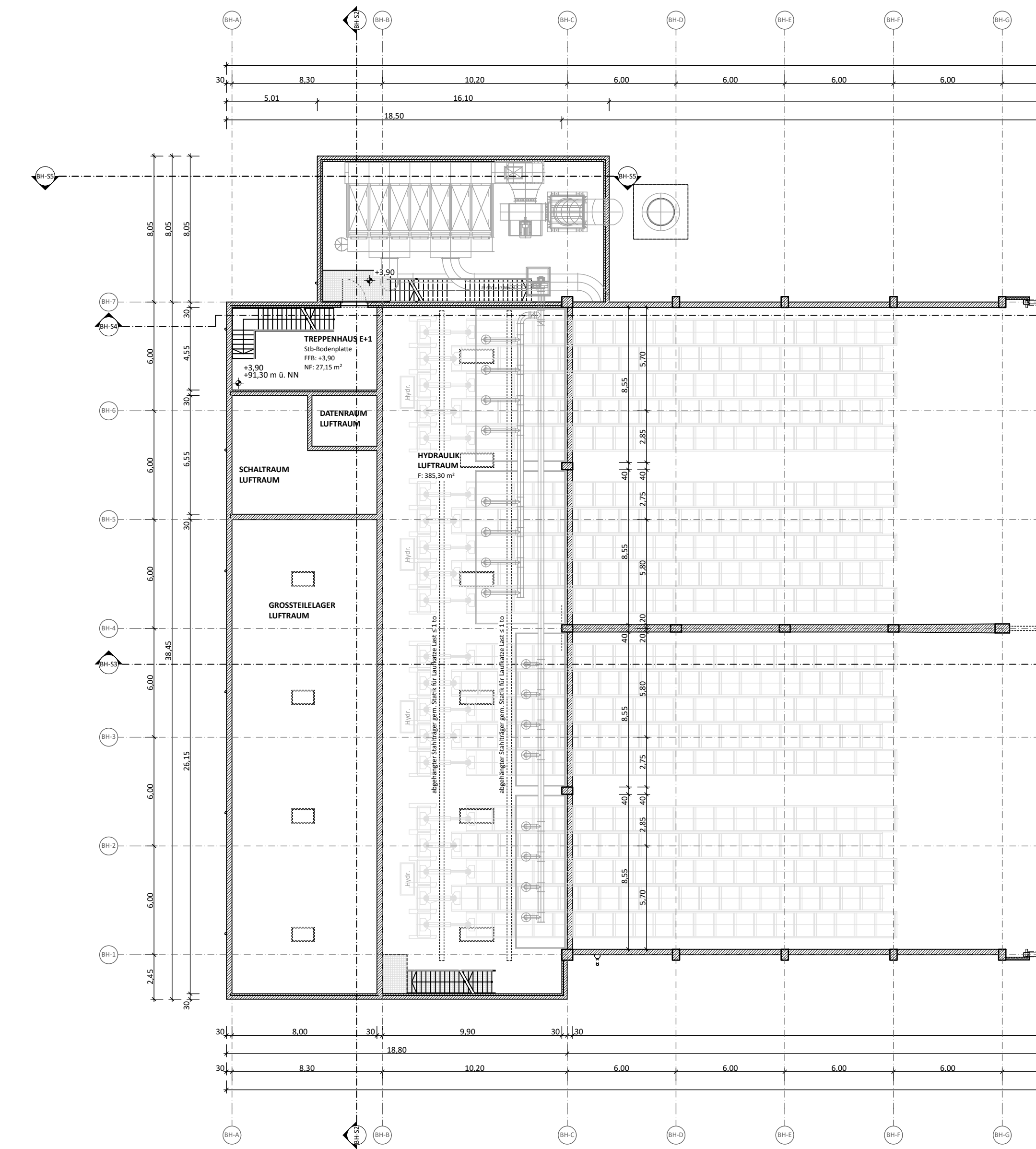
BRENNSTOFFLAGERHALLE 1. OBERGESCHOSS
