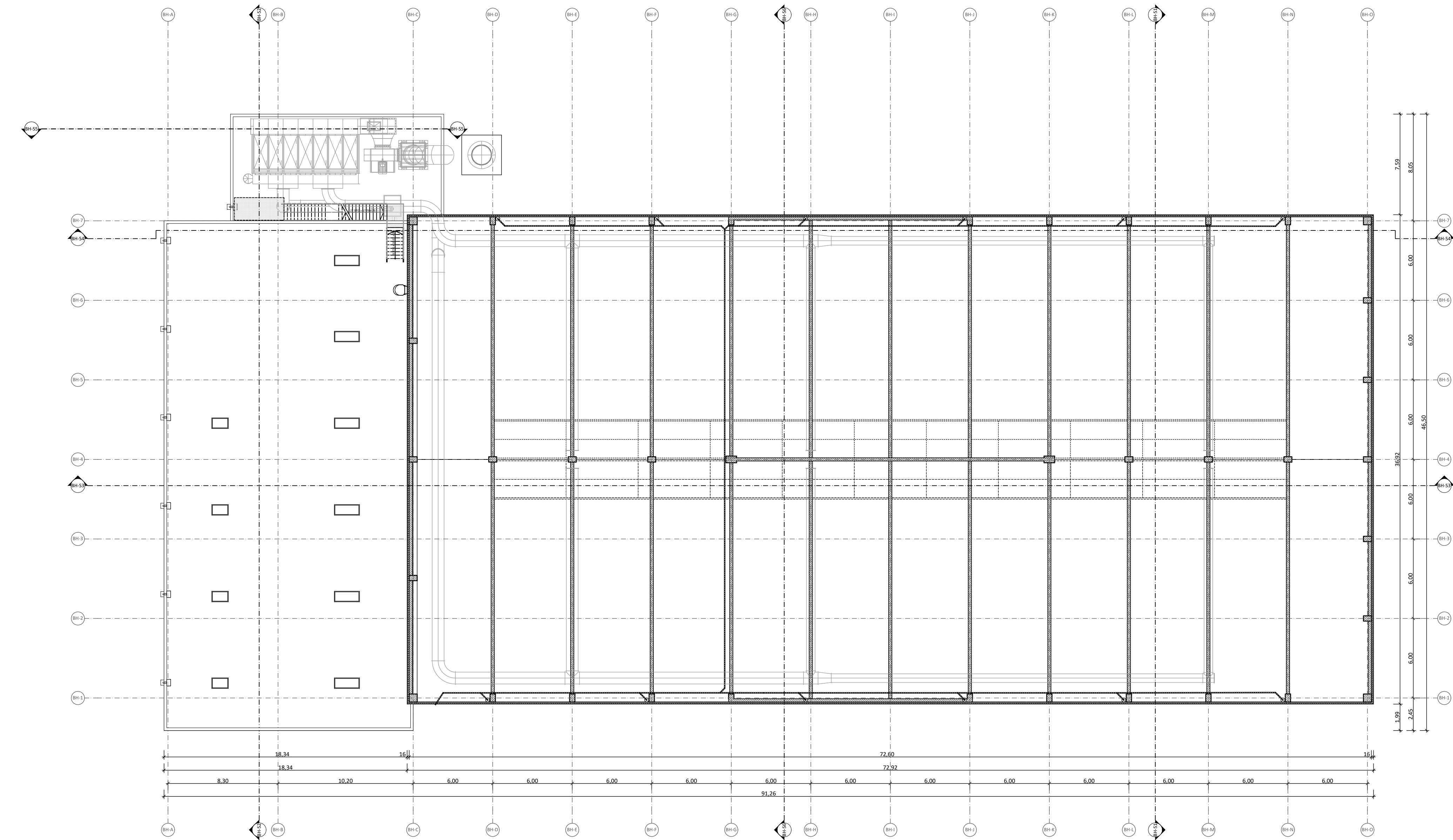
BRENNSTOFFLAGERHALLE 2. OBERGESCHOSS
