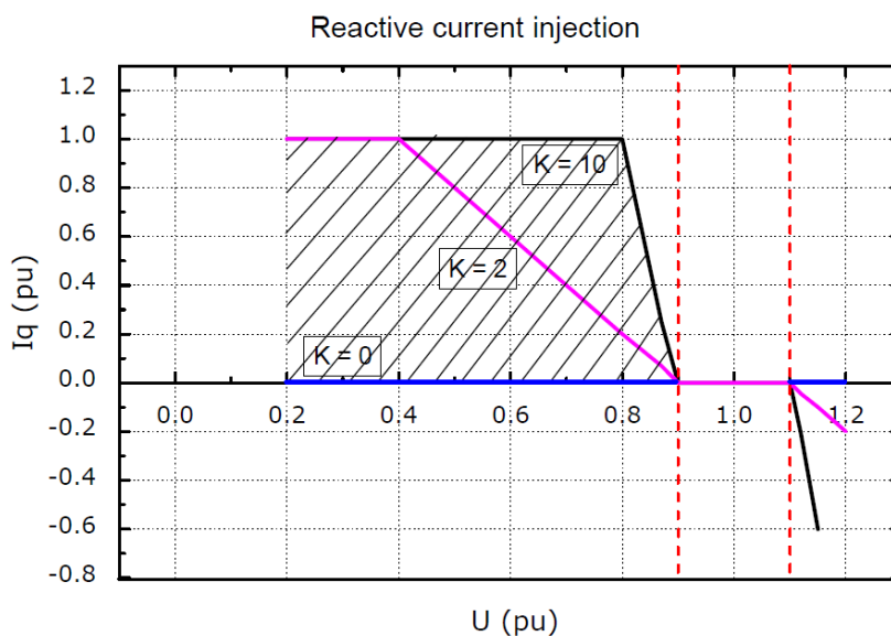
Abbildung 10-11: Blindstromeinspeisung.
