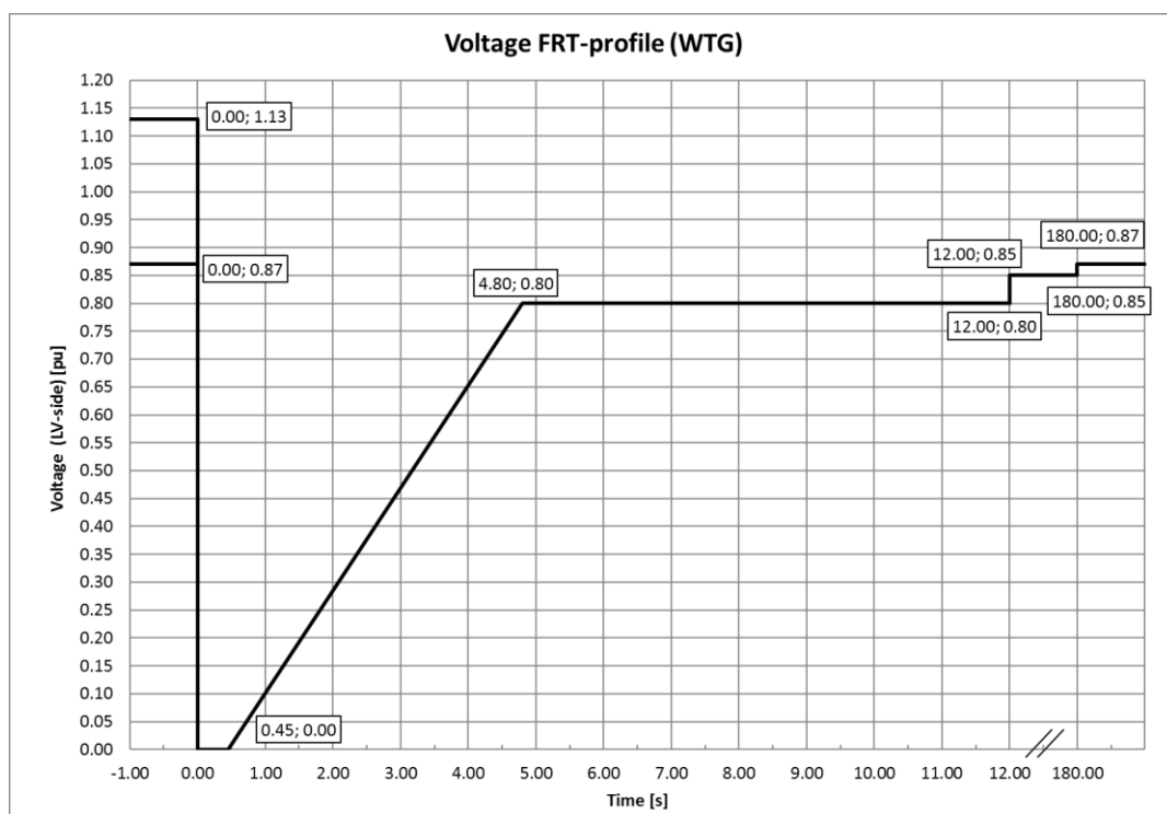
Abbildung 10-10: Niedrige Spannungstoleranzkurve für symmetrische und asymmetrische Störungen, wobei U die gemessene Spannung im Stromnetz darstellt.
