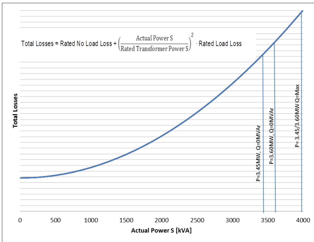
Abbildung 4-1: Gesamtverluste gegenüber tatsächlicher Leistung.
