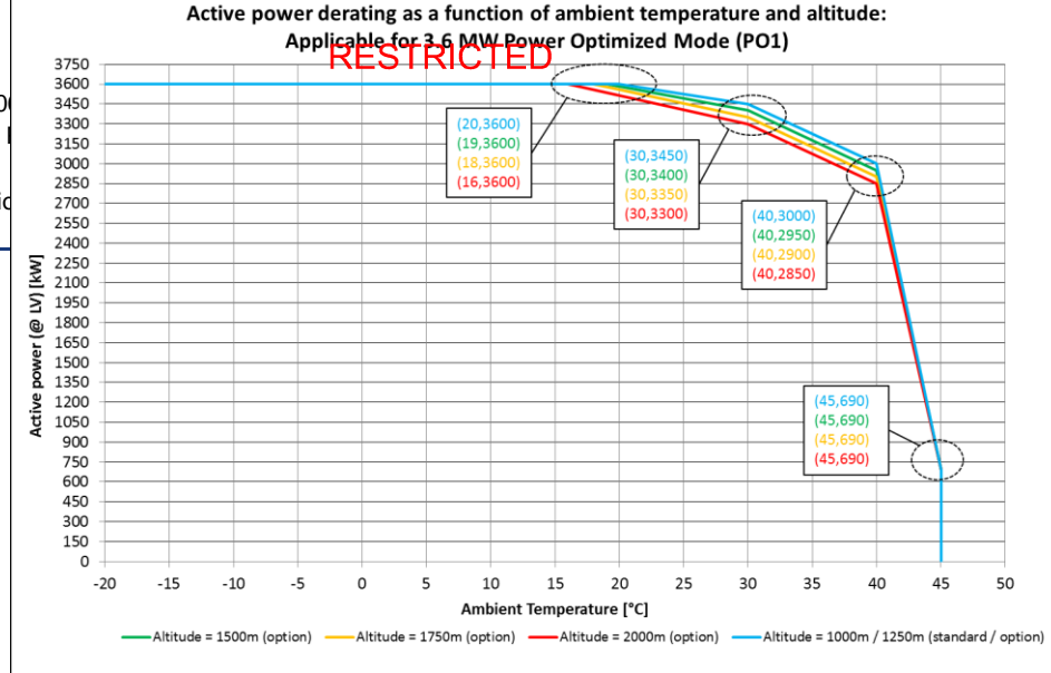
Abbildung 10-2: Temperatur- und höhenbedingter Teillastbetrieb im leistungsoptimierten 3,6-MW-Modus (PO1).
