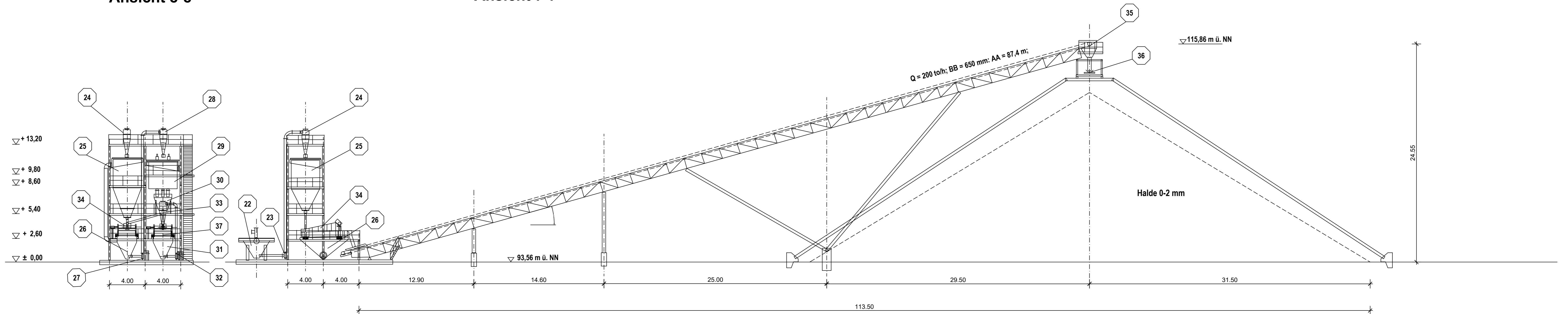
Ansicht 7-7
