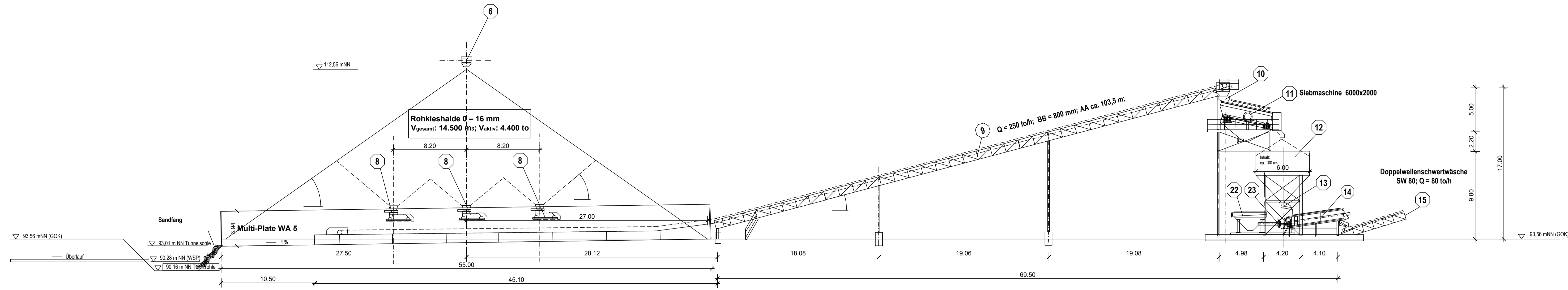
Ansicht 4-4
