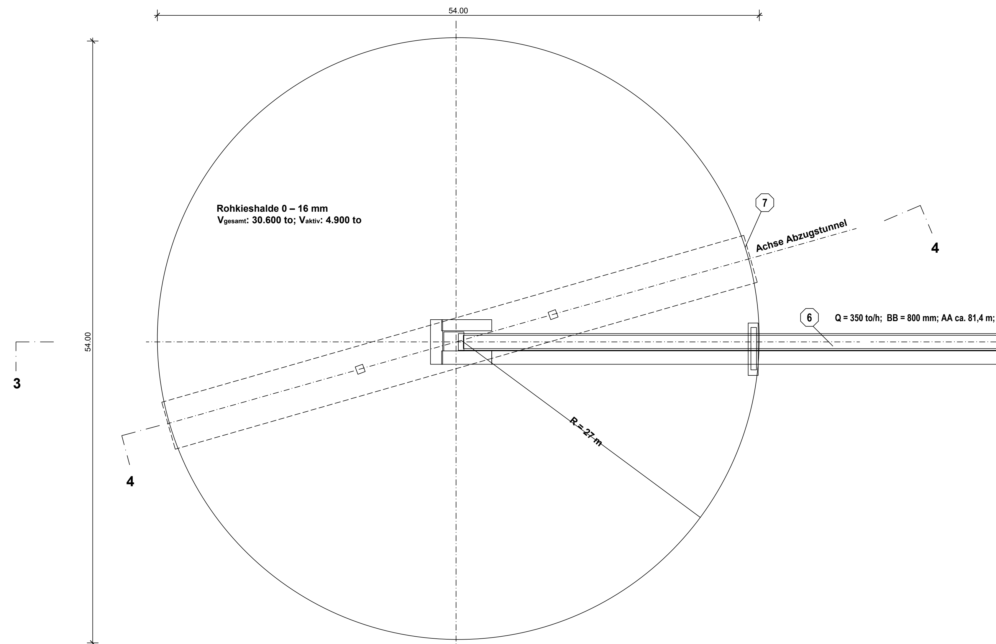
Grundriß Rohkieshalde
