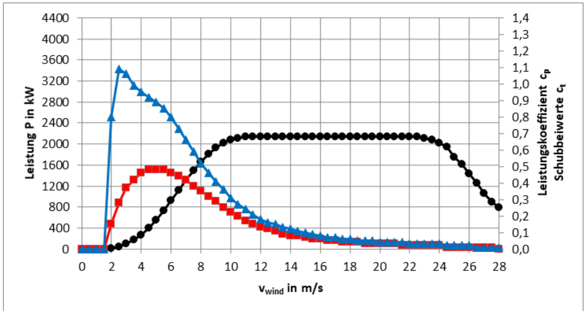
Abb. 1: Leistungs-, c_p - und c_t -Kennlinie E-138 EP3 E2 / 4200 kW Betriebsmodus NR 8
