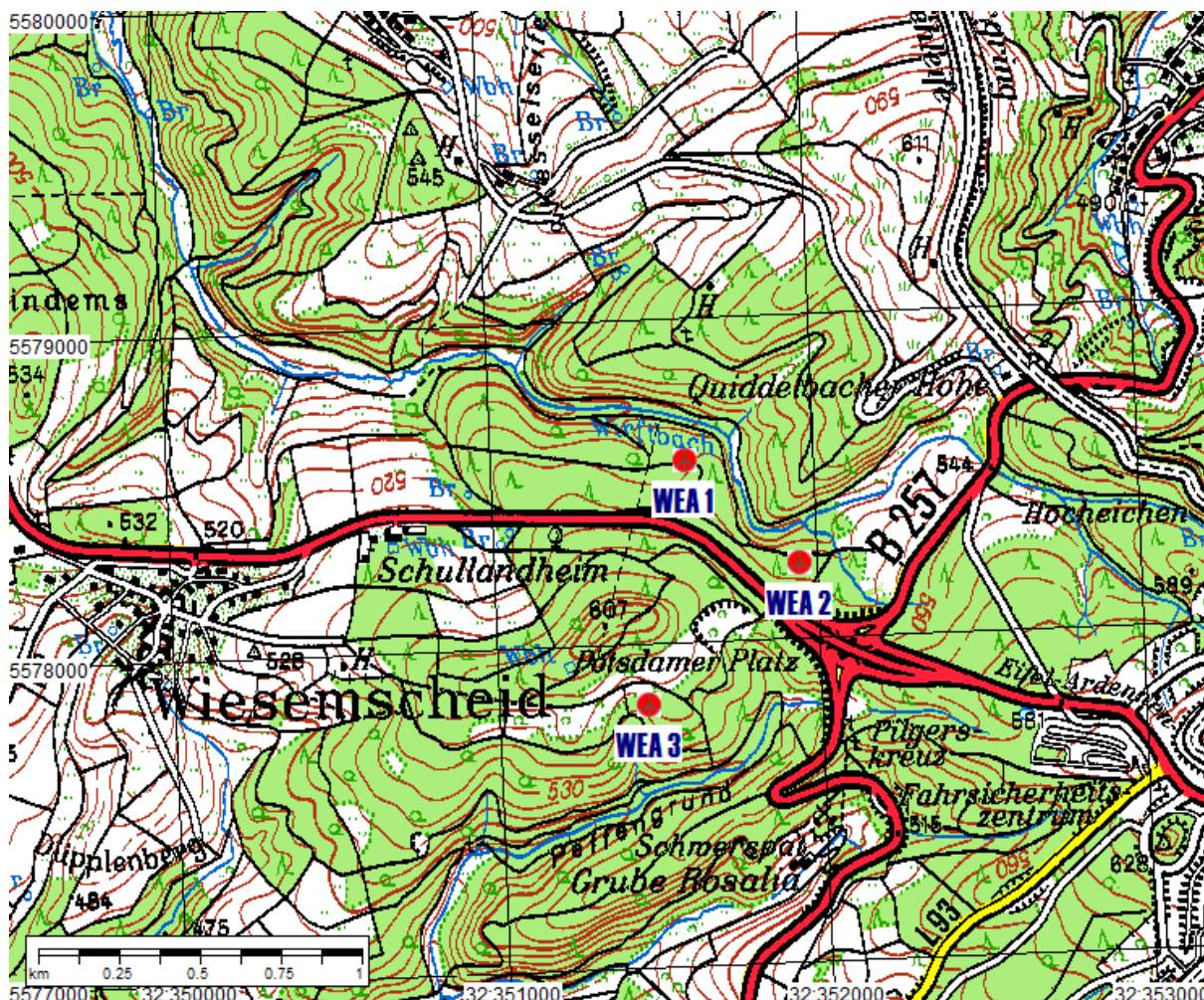
Abbildung 1: Lage des Windparks, Auszug topografische Karte 1:50.000 (vergrößerte Darstellung) /17/
