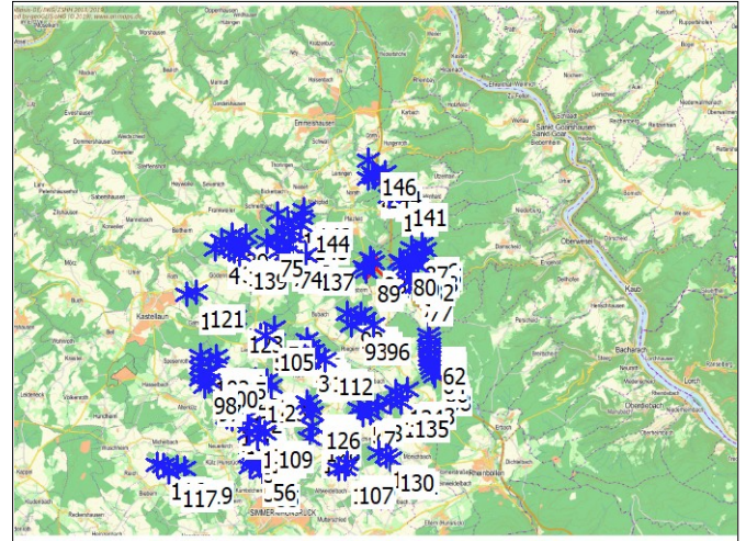
Maßstab 1:400.000 ★ Neue WEA ★ Existierende WEA
