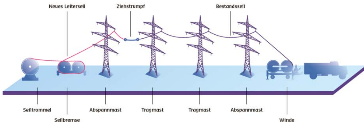
Abbildung 5: Prinzipdarstellung eines Seilzuges bei einer Umbeseilung (Quelle: Amprion GmbH)
