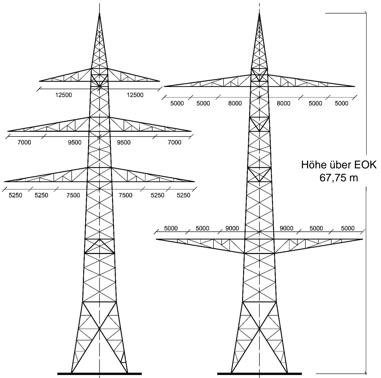
Schemazeichnung (ohne Maßstab) Maßangaben in Millimeter
