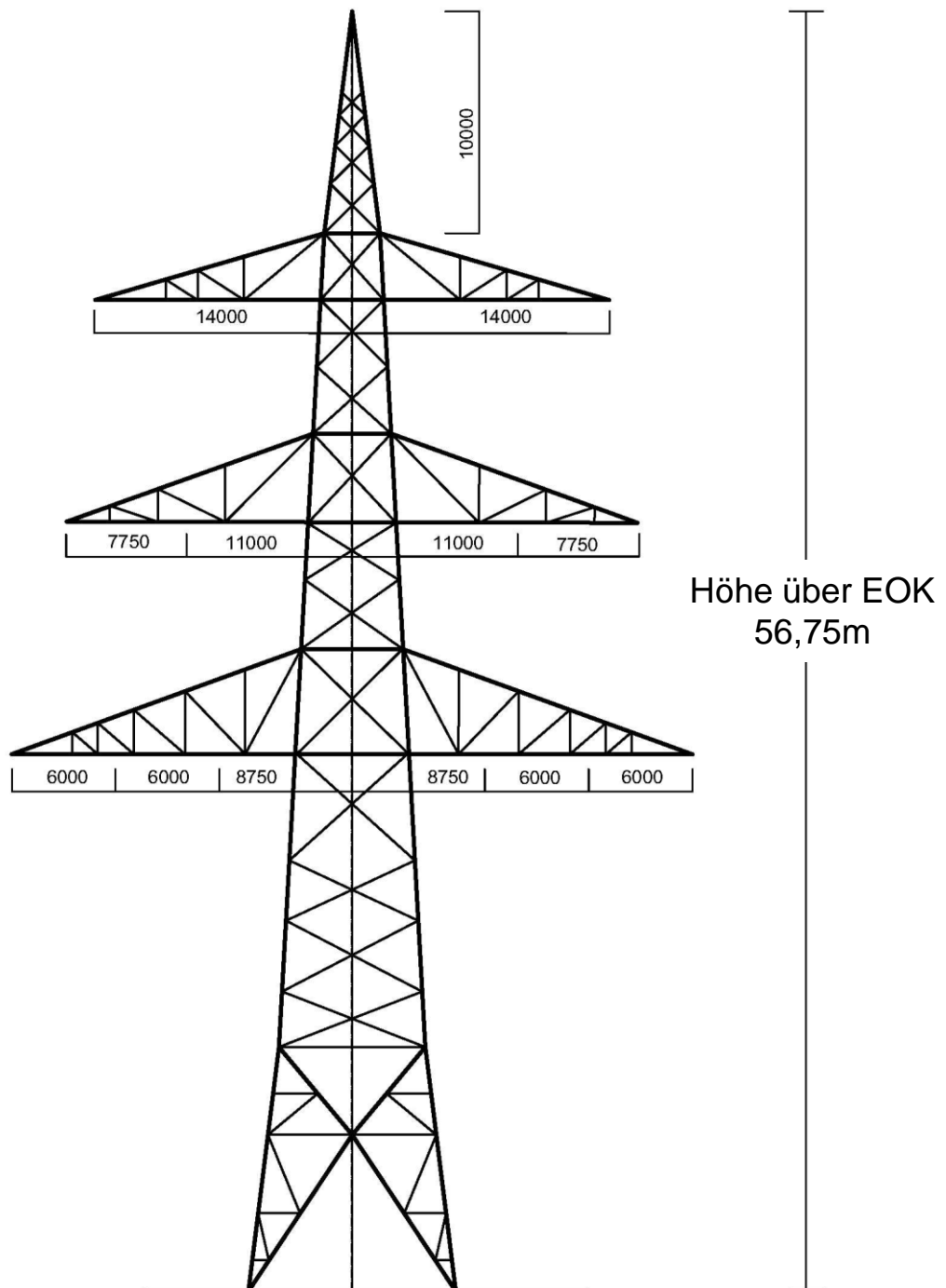
Schemazeichnung (ohne Maßstab) Maßangaben in Millimeter
