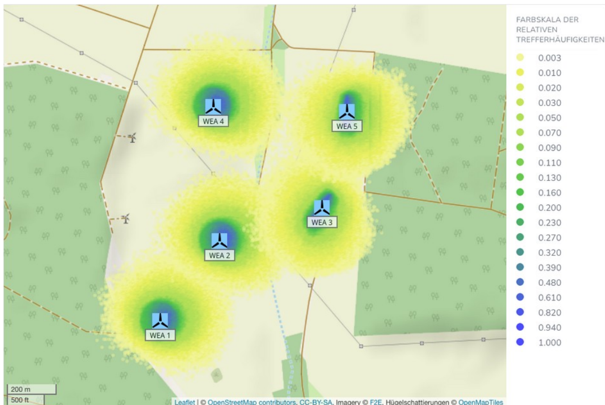
Abbildung A.1.1: Trefferhäufigkeiten von Eisstücken pro Rasterfläche (16m 2 ) und Jahr in der Umgebung der WEA 1 - 5 am Standort Fürstenberg für eine Azimut-Position nach Abschaltung durch die Eiserkennung für die WEA 3 von 305° und für die WEA5 von 275° (Karte /1.4/).
