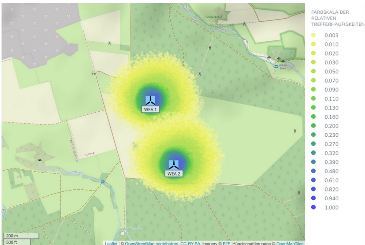
Abbildung A.1.1: Trefferhäufigkeiten von Eisstücken pro Rasterfläche (16m 2 ) und Jahr in der Umgebung der WEA 1 und 2 am Standort Warstein Altes Feld (Karte 1/1.4/).
