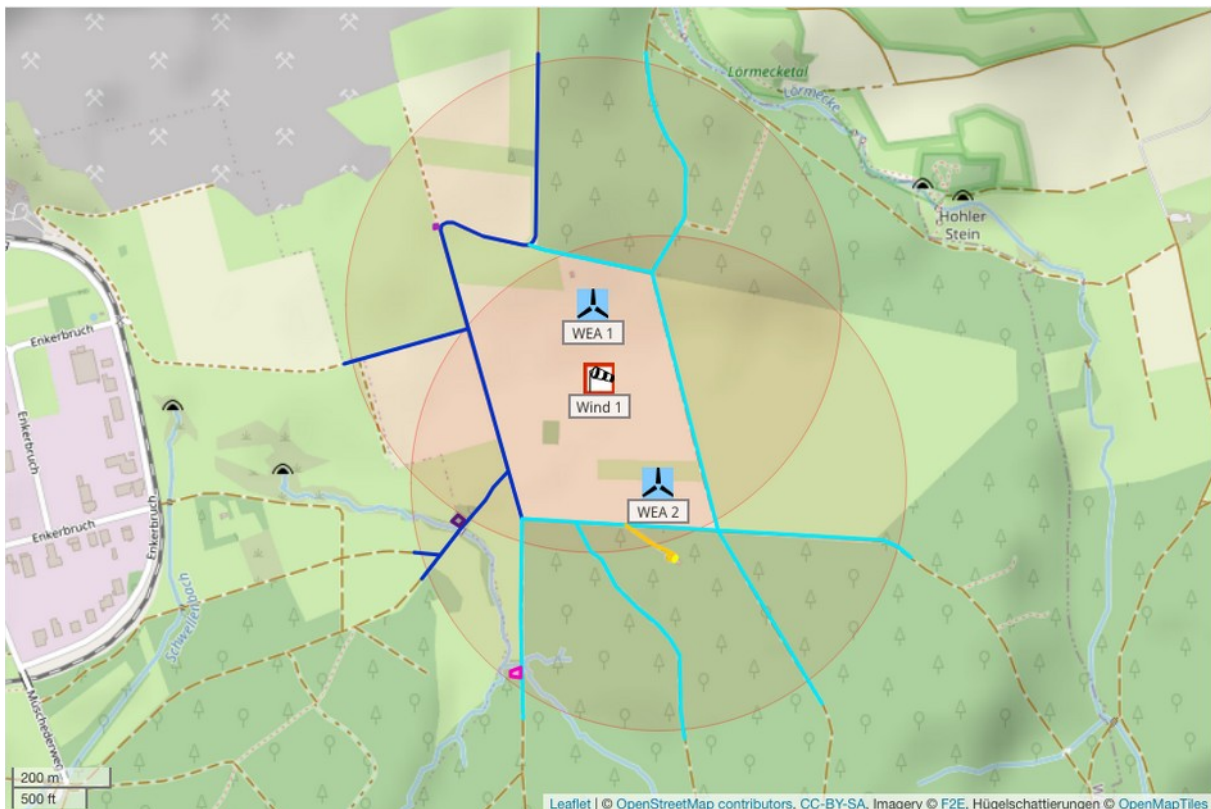
Abbildung 4.3.1: Potentielle Gefährdungsbereiche der WEA und Schutzobjekte am Standort Warstein Altes Feld (Karte /1.4/).
