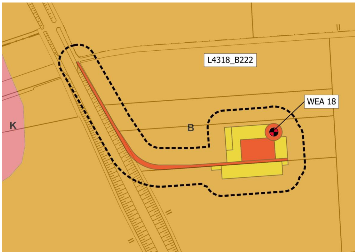
Abb. 1 Lage der geplanten Windenergieanlage WEA 18 (rot-schwarzer Kreis) und der Nutzflächen (rot = dauerhaft, gelb = temporär) zu den anstehenden Bodentypen gem. Bodenkarte BK 50 (WMS-FEATURE 2024) im Untersuchungsgebiet 25 m (schwarze Strichlinie).
