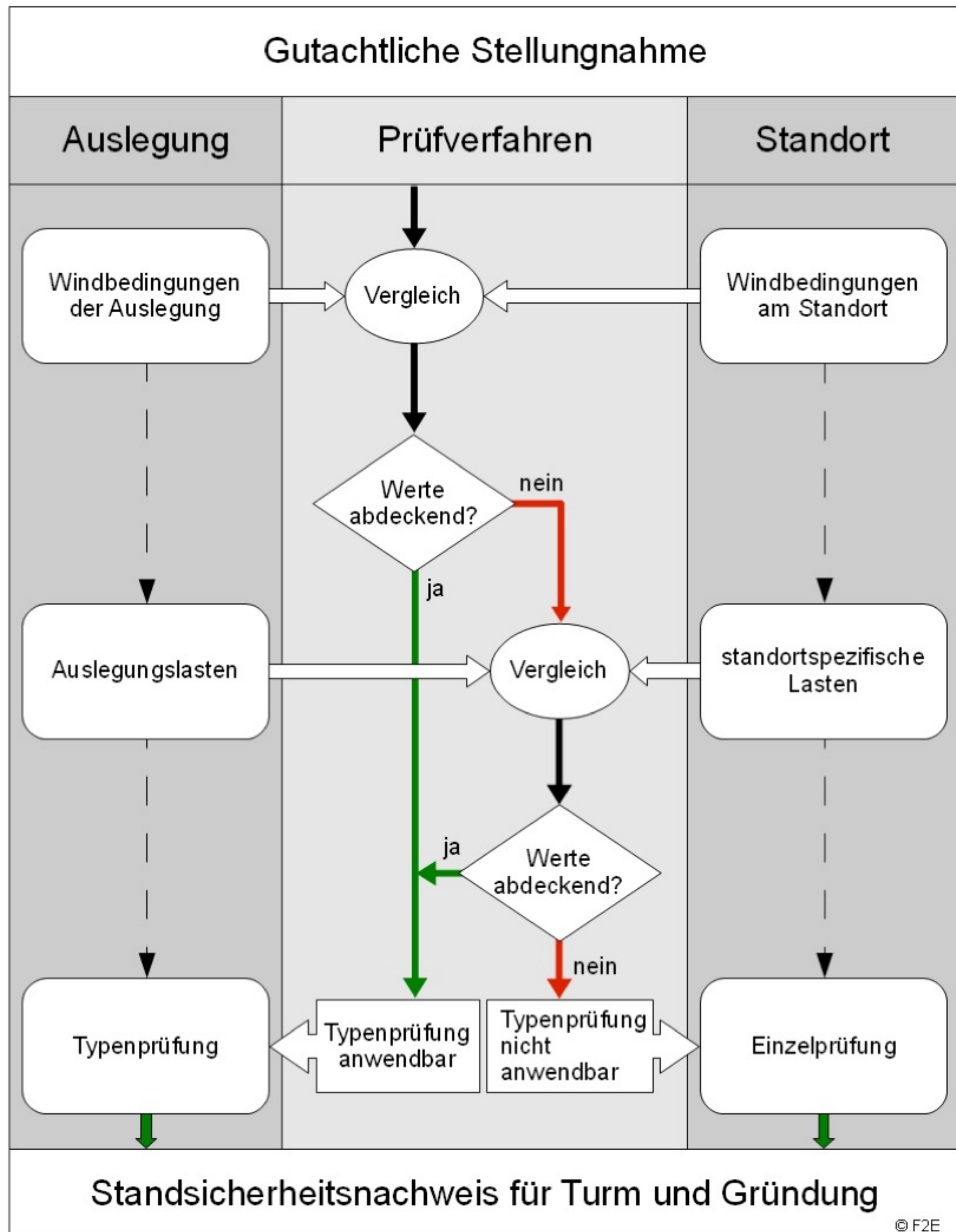
Abbildung 2.1.1: Schematische Darstellung des Prüfverfahrens.
