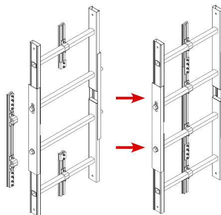
Flanschverbindingssatz
