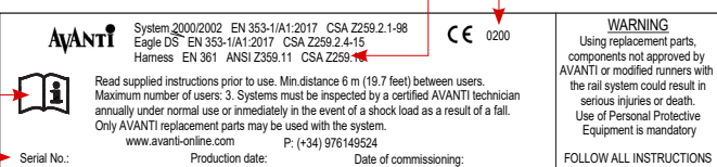
Typenschild der Sicherheitsschiene
