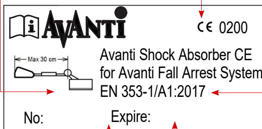
Etikett des Falldämpfers
