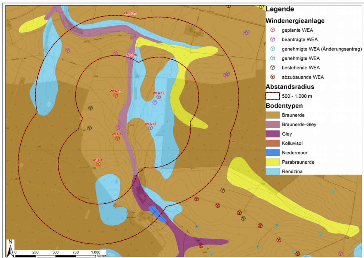
Abbildung 5: Auszug aus der Bodenkarte 1:50.000 des GeoPortals NRW (Zugriff am: 08.12.2022). Eigene Bearbeitung.
