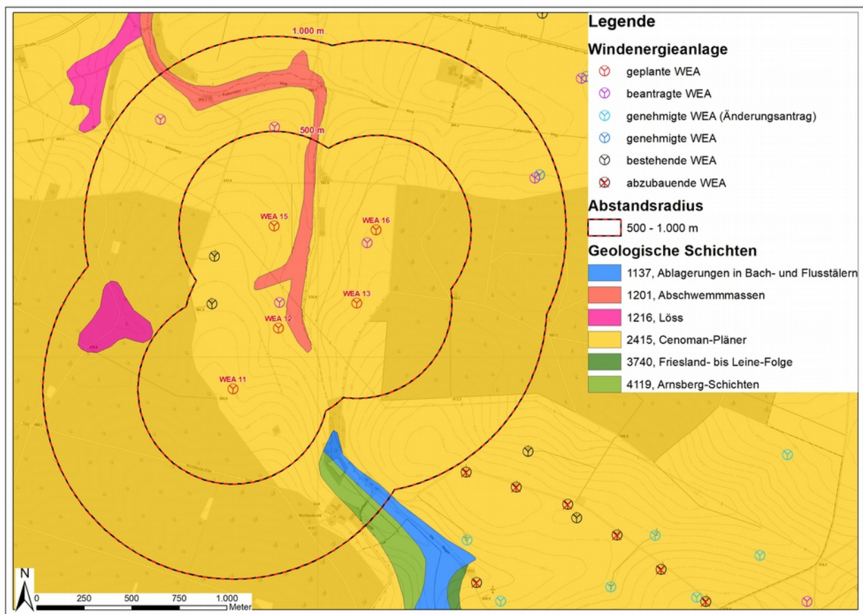
Abbildung 4: Auszug aus der Geologischen Karte 1:100.000 des GeoPortals NRW (Zugriff am: 08.12.2022). Eigene Bearbeitung.
