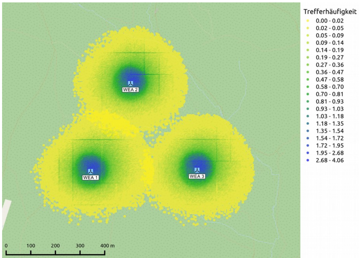
Abbildung A.1.1: Trefferhäufigkeiten von Eisstücken pro Rasterfläche (16m 2 ) und Jahr in der Umgebung der WEA 1 - 3 am Standort Freudenberg Kuhlenberg (Karte I/7).
