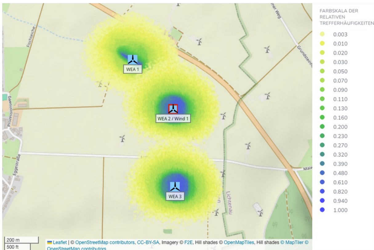
Abbildung A.1.1: Trefferhäufigkeiten von Eisstücken pro Rasterfläche (16m 2 ) und Jahr in der Umgebung der WEA 1 -3 für eine Azimut-Position nach Abschaltung durch die Eiserkennung für die WEA 1 von 210°.
