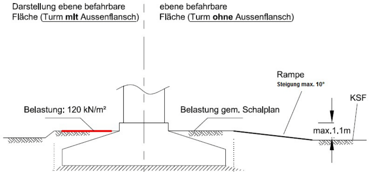
Abb. 22 Fläche um den Turm im Schnitt
