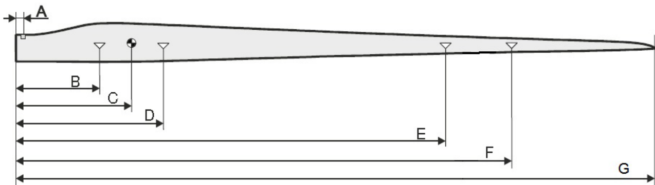
Abb. 5 Transportabmessungen Rotorblatt Seitenansicht
