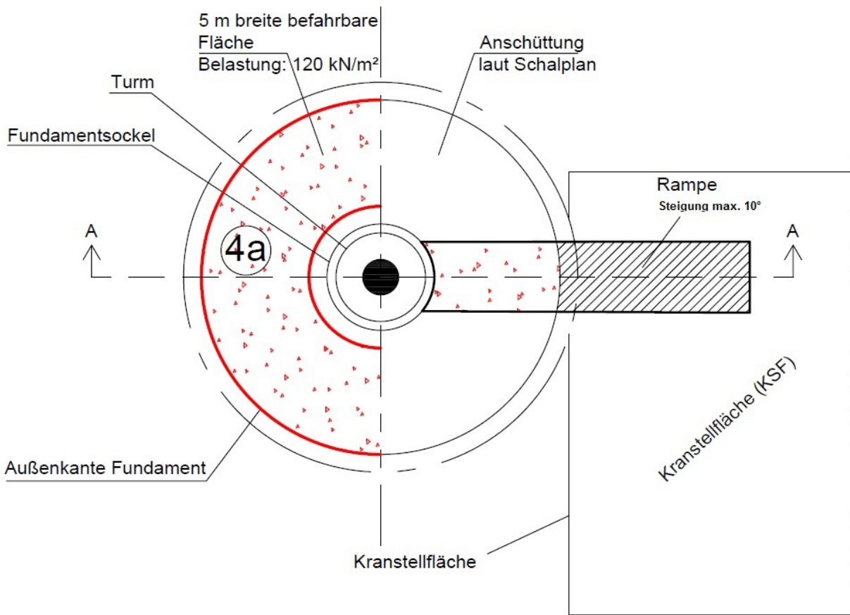
Abb. 23 Fläche um den Turm in Draufsicht (Stahlrohrturm)
