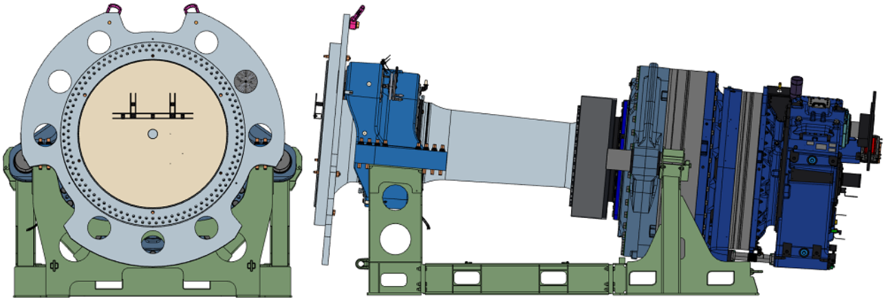
Abb. 3 Triebstrang auf Transportvorrichtung, Ansicht von vorn und von links
