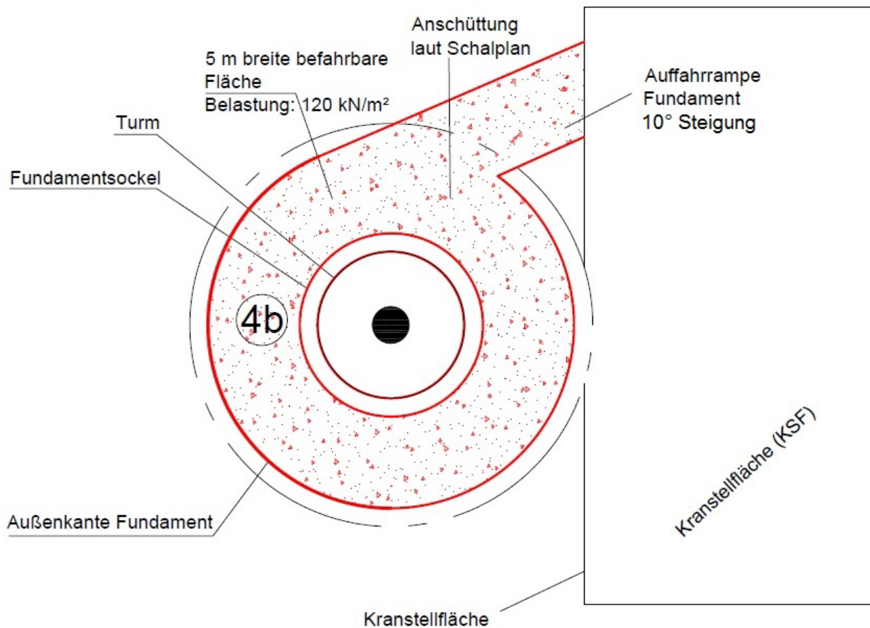
Abb. 24 Fläche um den Turm in Draufsicht (Hybridturm)
