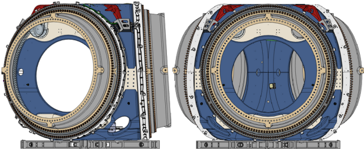
Abb. 4 Rotornabe auf Transportgestell; Ansicht von vorn und links aus der Transportrichtung
