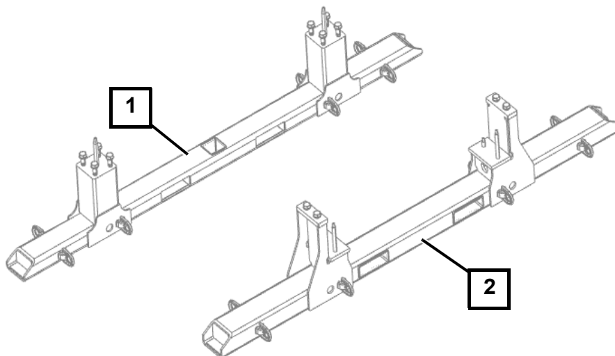
Abb. 7 Transportfüße Maschinenhaus vorn (1) und hinten (2)
