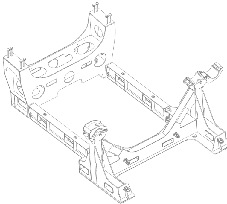
Abb. 8 Transportvorrichtung Triebstrang
