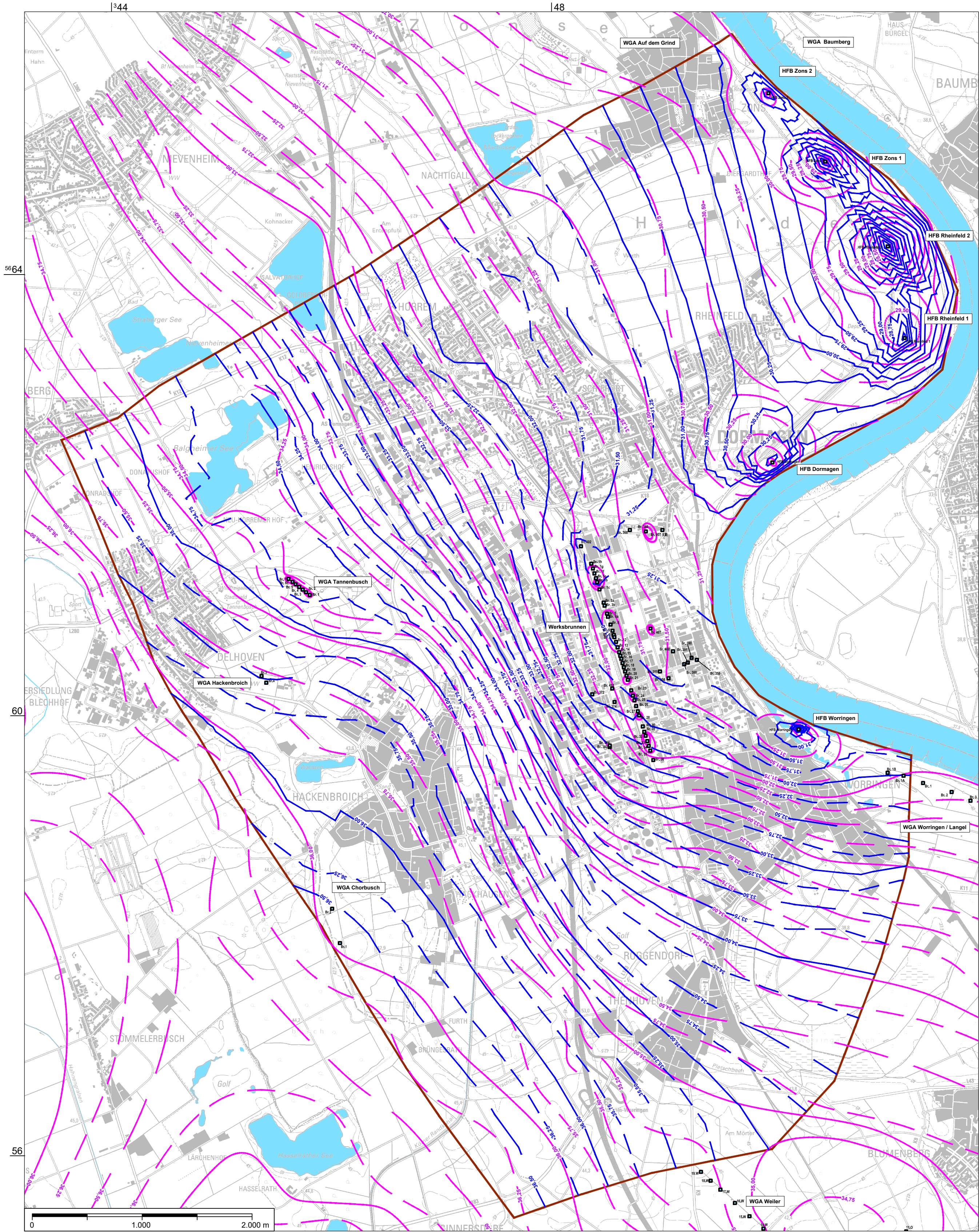
Grundwassergleichen 29.10.2018 (NW)
