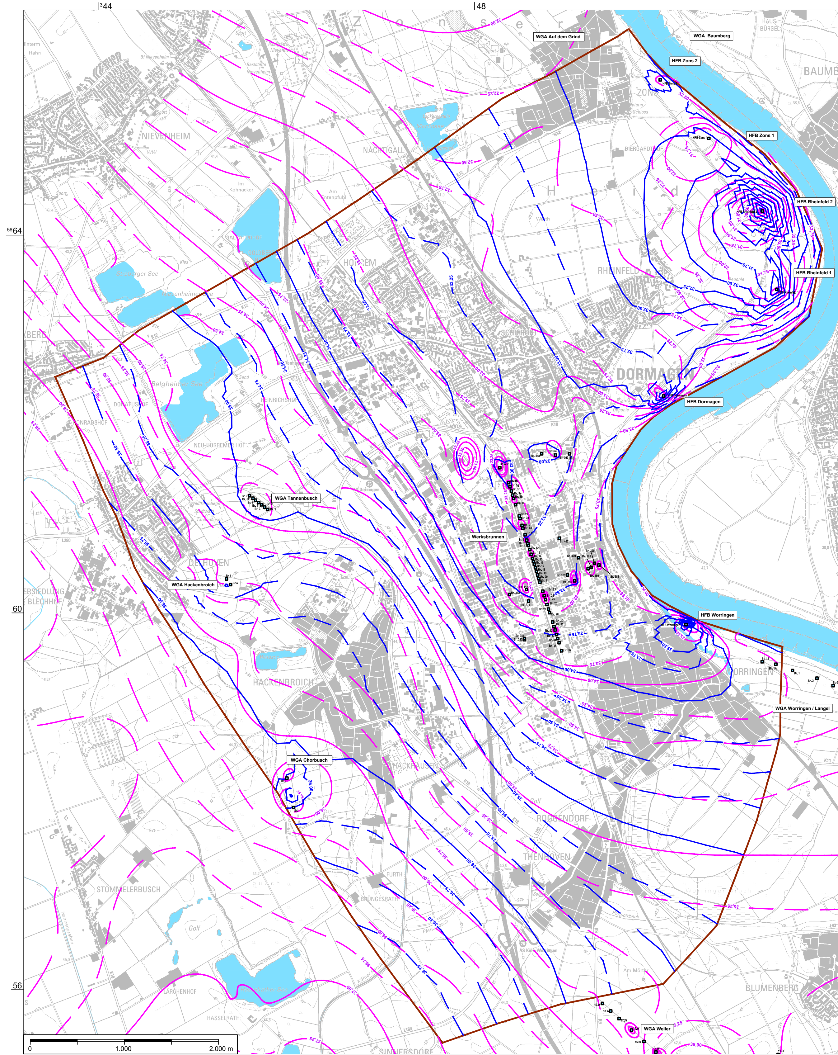
Grundwassergleichen 27.10.2014 (MW)
