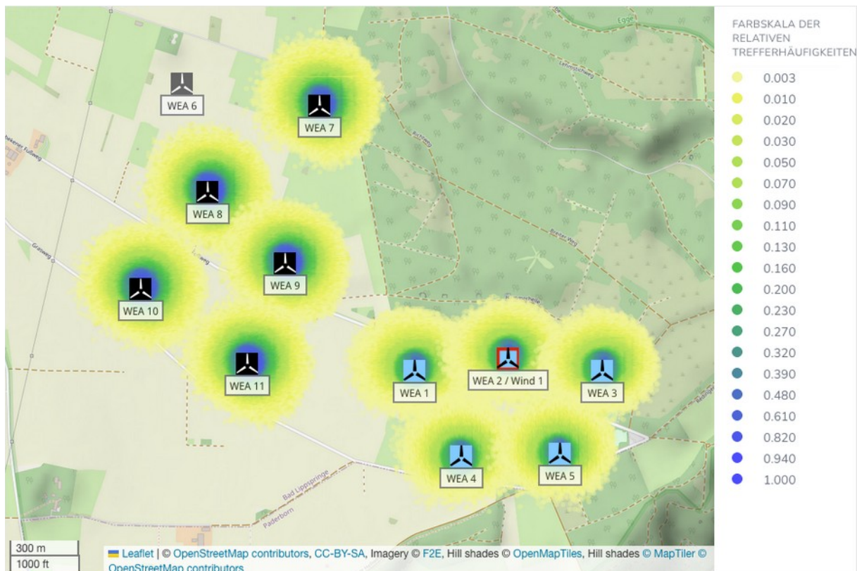
Abbildung A.1.1: Trefferhäufigkeiten von Eisstücken pro Rasterfläche (16m 2 ) und Jahr in der Umgebung der WEA 1 – 5 und 7 – 11.
