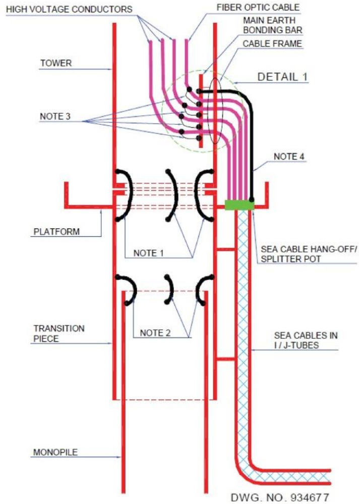
Abbildung 3-11: Prinzipdarstellung des Vestas-Erdungssystems bei J-Rohr-Aufstellung
