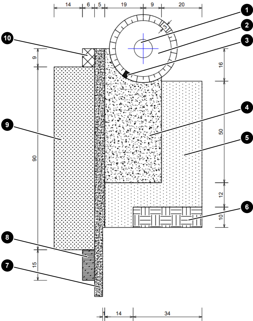
Abb. 14: Alternativer Arbeitsbereich am WEA-Standort, Baumaß (alle maßangaben in Meter)
