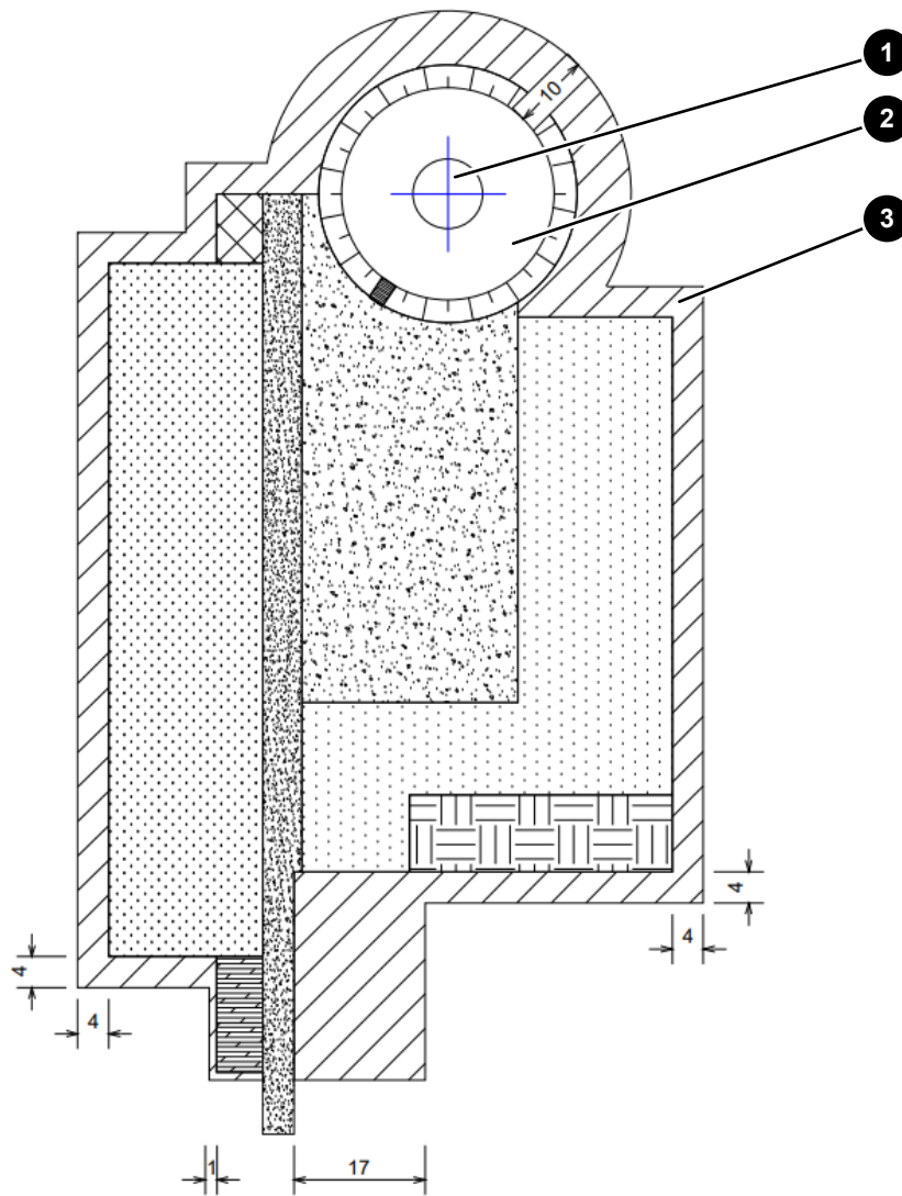
Abb. 15: Alternativer Rodungs- und Sicherheitsbereich, Baumaß (alle Maßangaben in Meter)
