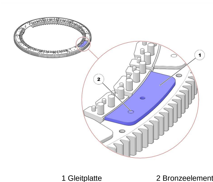
Abbildung 3-5 Darstellung eines Azimutlagerschutzes
