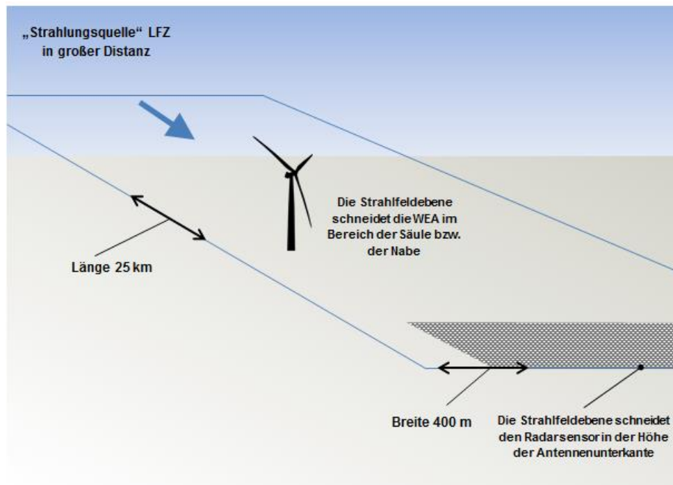
Abbildung 3: Anordnung von Radar und WEA sowie Lage des in dieser Untersuchung dargestellten Luftraums mit einer Ausdehnung von (hier) 25 km x 400 m Breite. Das Lfz wird in einer Distanz von bis zu 130 NM angenommen. – schematische Darstellung –
