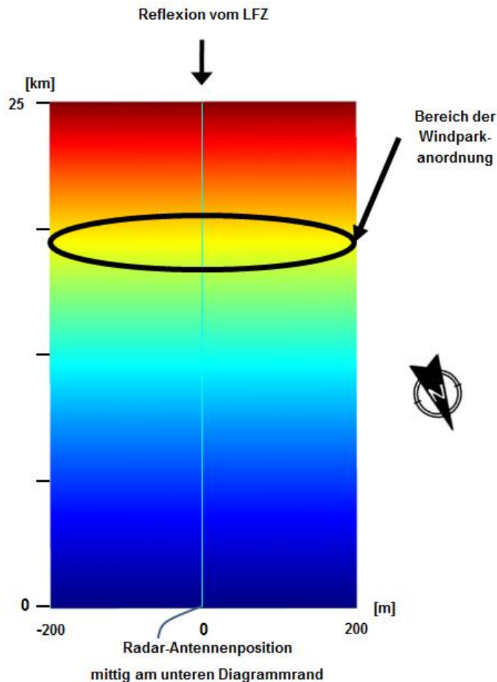
Abbildung 4: Feldgebiet von 25 km x 400 m in der Übersicht (schematische Übersicht für das Radar Erndtebrück)
