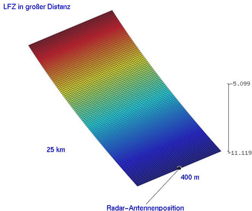
Abbildung 5: Das dargestellte Raumgebiet mit einer Elevation von -0,1^\circ ohne WEA-Einfluss in der Konturdarstellung für die Betriebsfrequenz des Radars Erndtebrück
