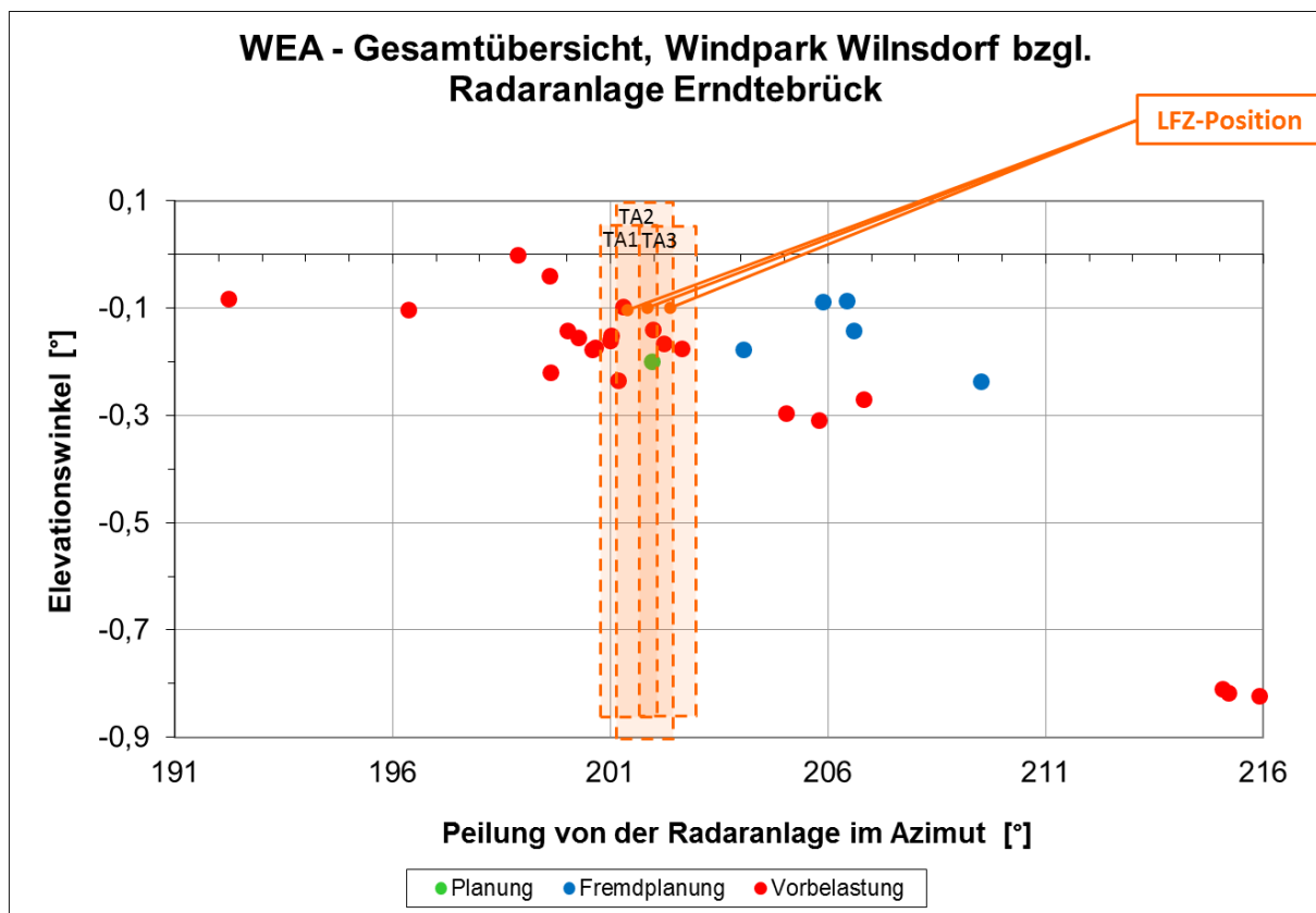
Abbildung 10: Perspektive zur Gondelanordnung gemäß Azimut und Elevation für die Position des Radars Erndtebrück. Die Bereiche der analysierten Teilanordnungen sind durch farbige Flächen gekennzeichnet. Die Richtung und Elevation des angenommenen Lfz ist dargestellt.
