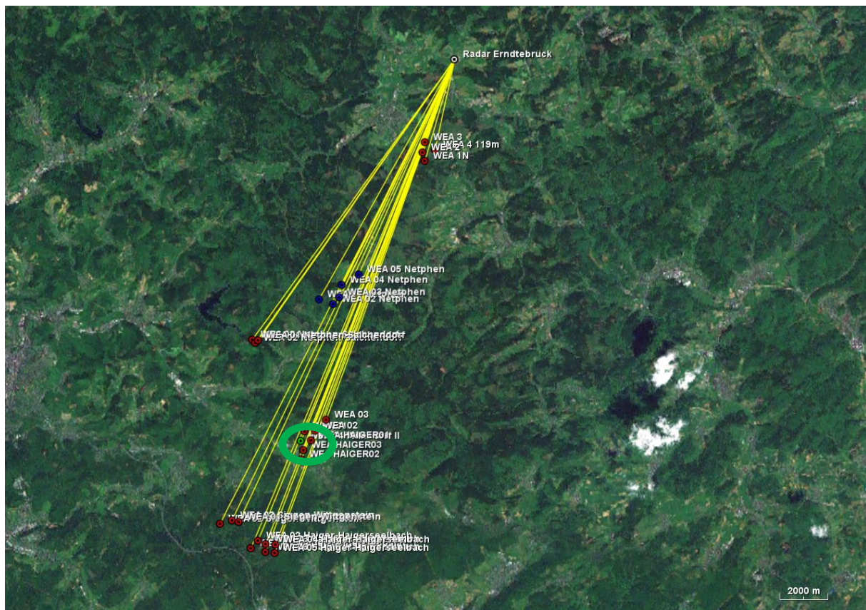
Abbildung 2: Luftaufnahme des Windparks Wilnsdorf mit der geplanten Windenergieanlage (grün), der Fremdplanung (blau) sowie der relevanten Vorbelastung (rot). Die Einstrahlungsrichtungen bzgl. der Radaranlage Erndtebrück sind gelb dargestellt. Um eine bessere Übersicht zu gewährleisten wurden die Bezeichnungen von einzelnen Anlagen teilweise ausgeblendet.
