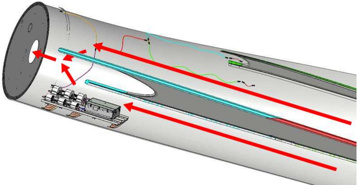
Abbildung 7.21: Evakuierungsroute im Blatt zur Nabe (V162 VAS)
