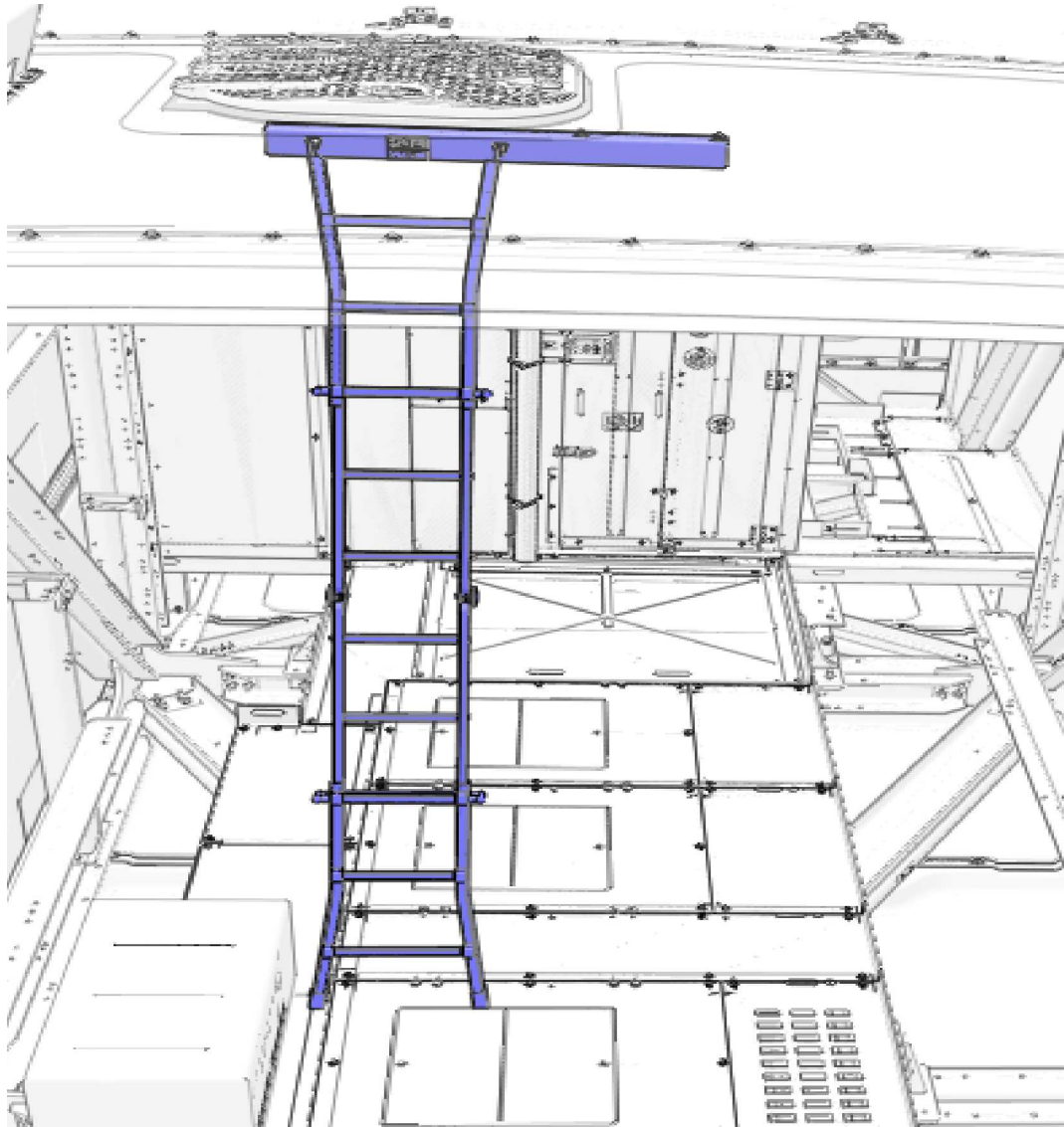
Abbildung 7.10: Tragbare Klappleiter
