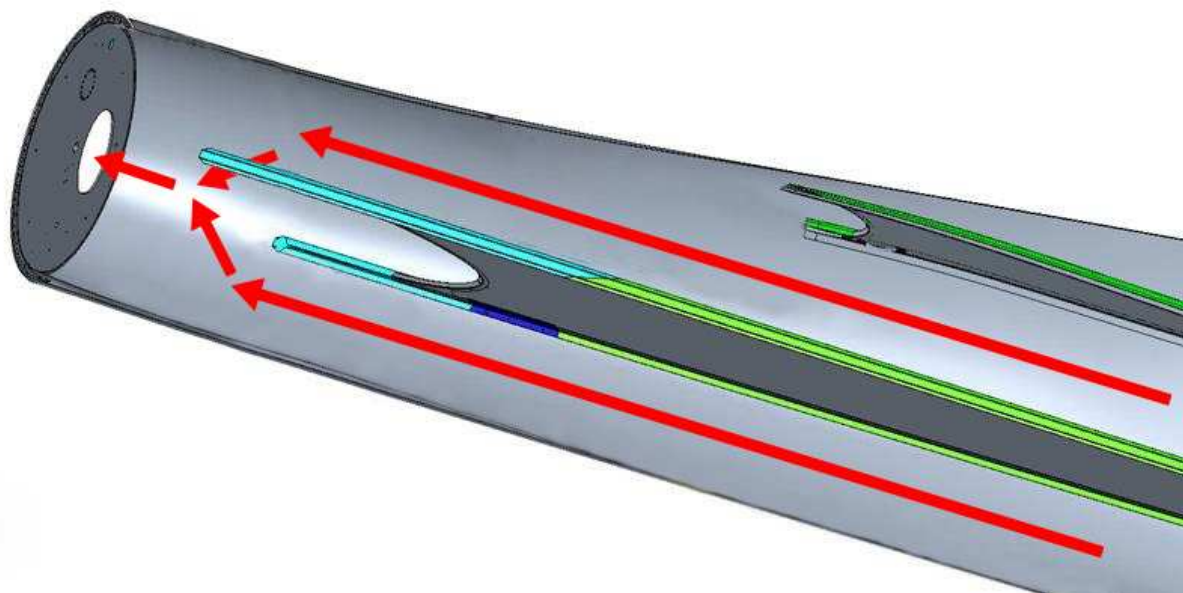
Abbildung 7.18: Evakuierungsrouten im Blatt zur Nabe (EnVentus™ V150-5.6 MW)
