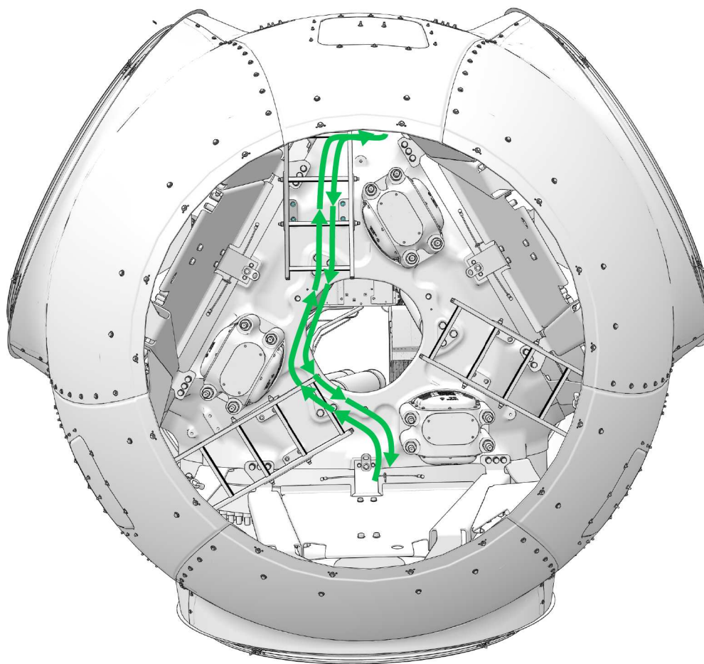
Abbildung 7.17: Zugang und Evakuierungsroute von der Nabe
