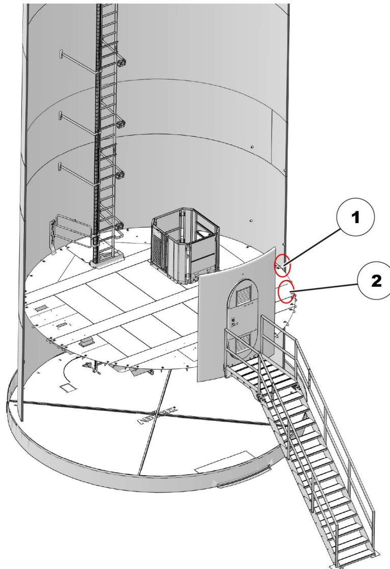
Abbildung 8.2: Standort der Sicherheitsausrüstung im Turm
