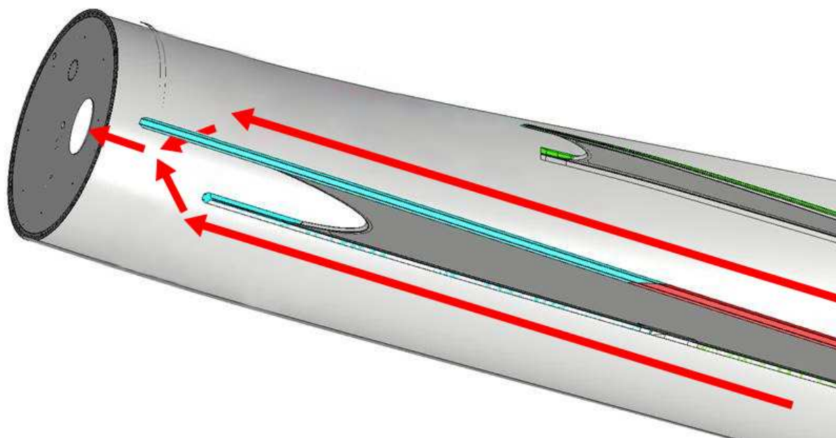
Abbildung 7.20: Evakuierungsroute im Blatt zur Nabe (EnVentus™ V162-5.6 MW)
