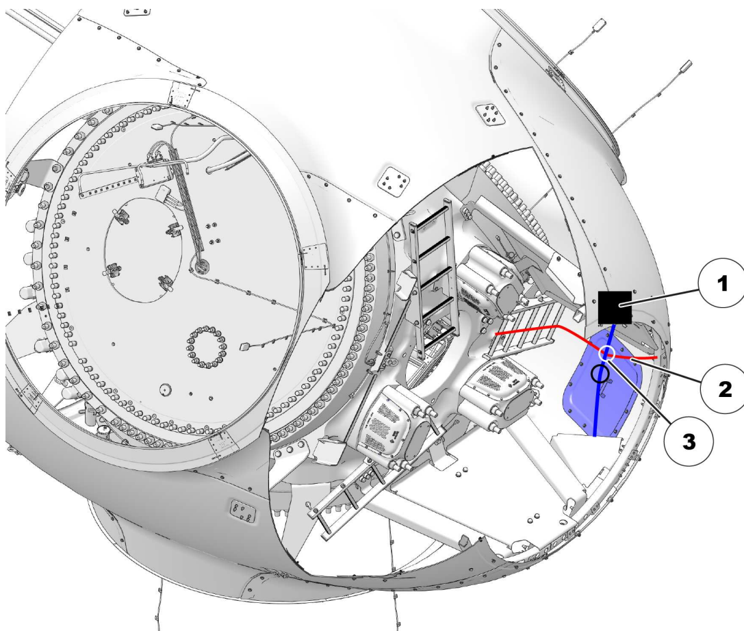
Abbildung 7.31: Geräteaufbau im Spinner
