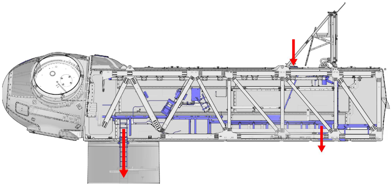
Abbildung 7.33: Rettungspunkte
