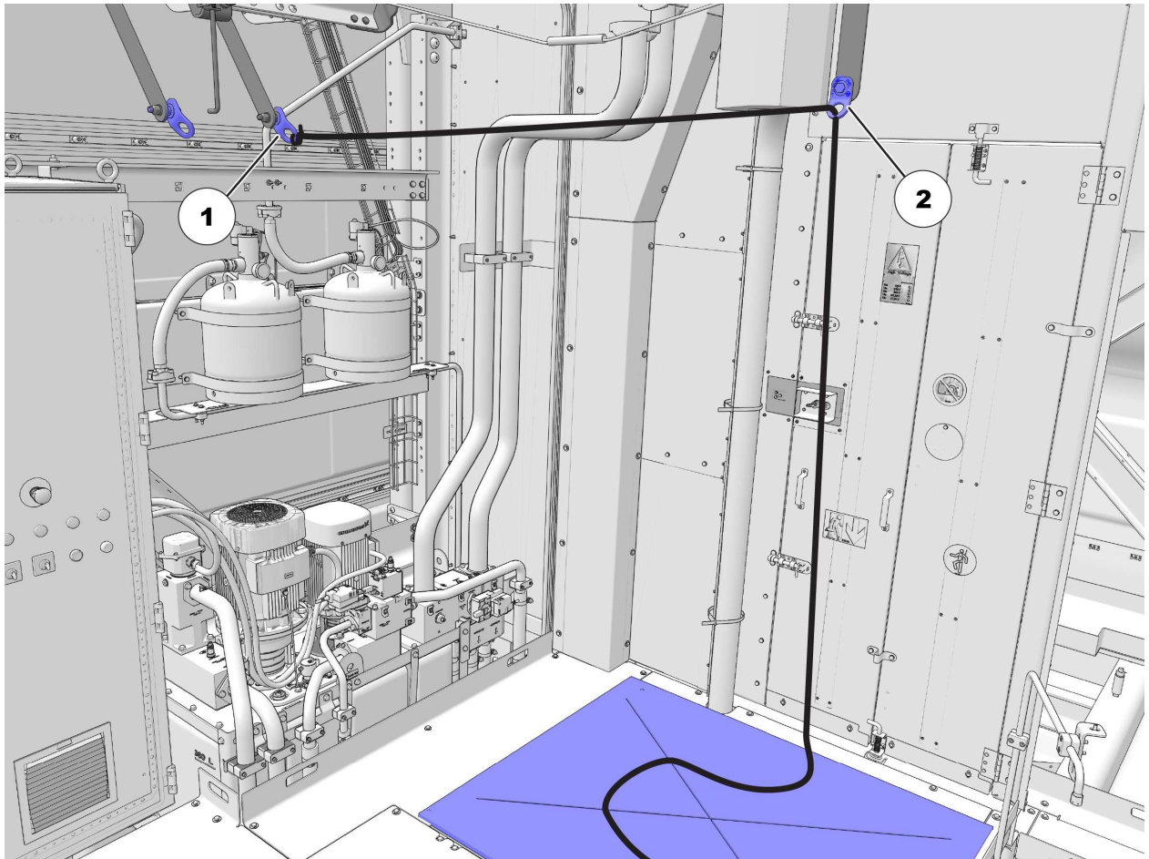
Abbildung 7.34: Aufbau der Abstiegsvorrichtung zum Absenken einer verletzten Person durch die Luke
