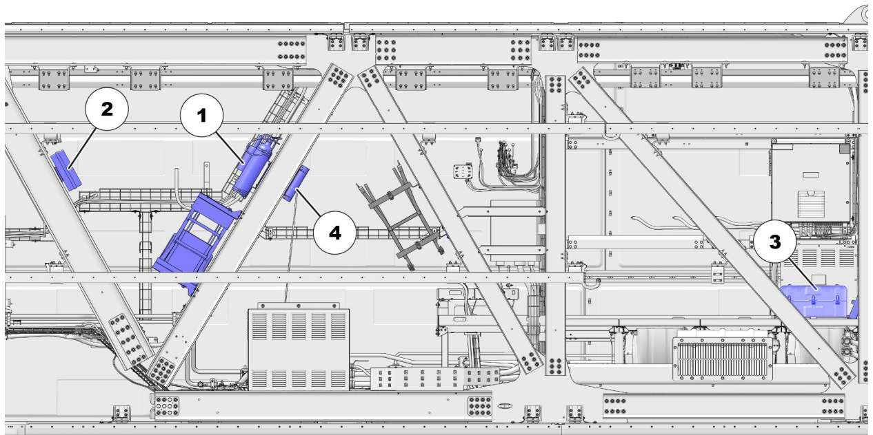
Abbildung 8.1: Sicherheitsausrüstung im Maschinenhaus
