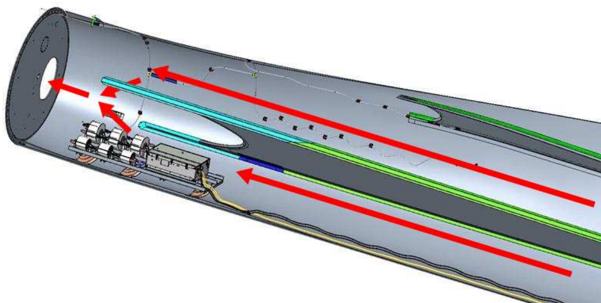
Abbildung 7.19: Evakuierungsroute im Blatt zur Nabe (V150 VAS)
