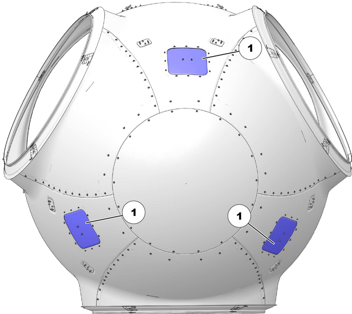
Abbildung 7.24: Luken im Spinner
