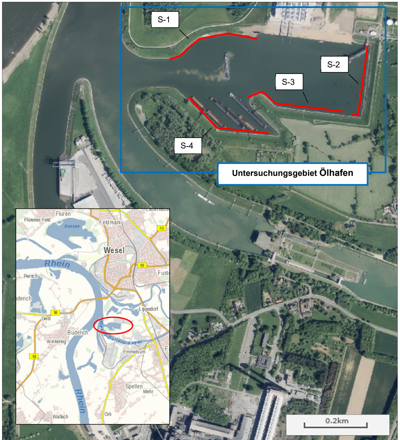
Abb. 1 Untersuchungsgebiet Ölhafen (Wesel) und Lage der Befischungstrecken S-1 – S-4 für die Elektrofischungen am 05.06.2019
