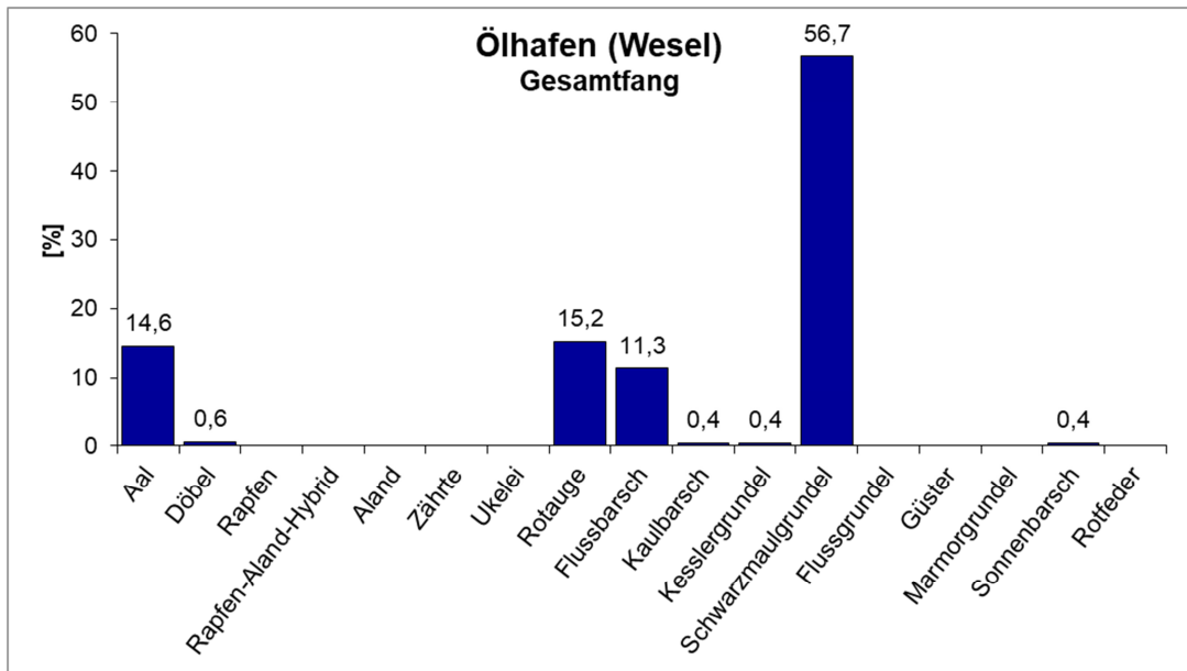
Abb. 3 Dominanzstruktur des Gesamtfangs (relative Häufigkeit der Arten in %) aus den Elektrofischungen im Ölhafen (Wesel) am 05.06.2019 (Arten angeordnet nach ökologischen Kriterien, Gesamtartenspektrum aus der Untersuchung von Ölhafen (Wesel) und Hafen Emmelsum)
