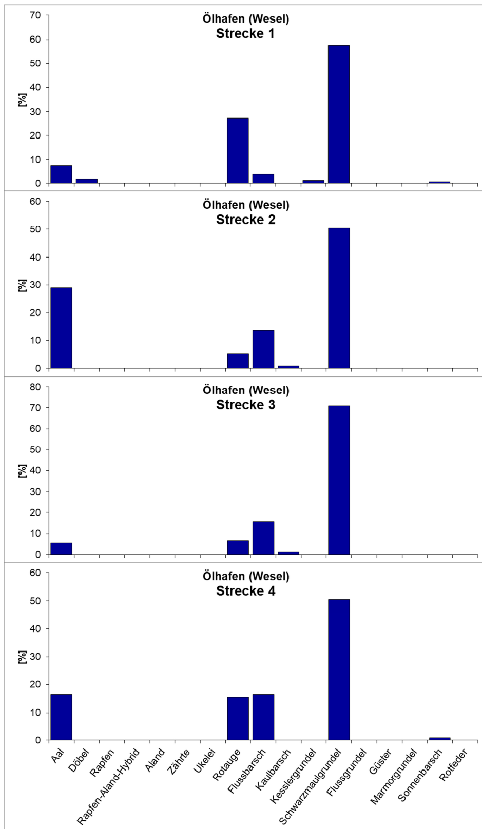
Abb. 5 Dominanzstruktur (relative Häufigkeit der Arten in %) der Teilfänge in den einzelnen Befischungsstrecken S1 – S4 (vgl. Abb. 1) der Elektrofischungen im Ölhafen (Wesel) am 05.06.2019 (Arten angeordnet nach ökologischen Kriterien, Gesamtartenspektrum aus der Untersuchung von Ölhafen (Wesel) und Hafen Emmelsum)
