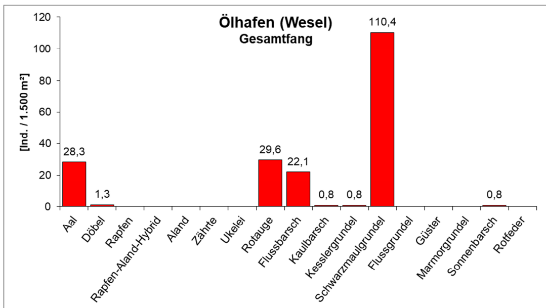
Abb. 4 Mittlere Individuendichten (Individuen pro 1.500 m 2 Befischungsfläche) der nachgewiesenen Fischarten bei den Elektrofischungen im Ölhafen (Wesel) am 05.06.2019 (Arten angeordnet nach ökologischen Kriterien, Gesamtartenspektrum aus der Untersuchung von Ölhafen (Wesel) und Hafen Emmelsum)
