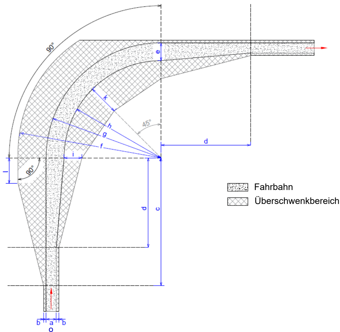
Abb. 2: 90-Grad-Kurve (Konstruktionsschema)
