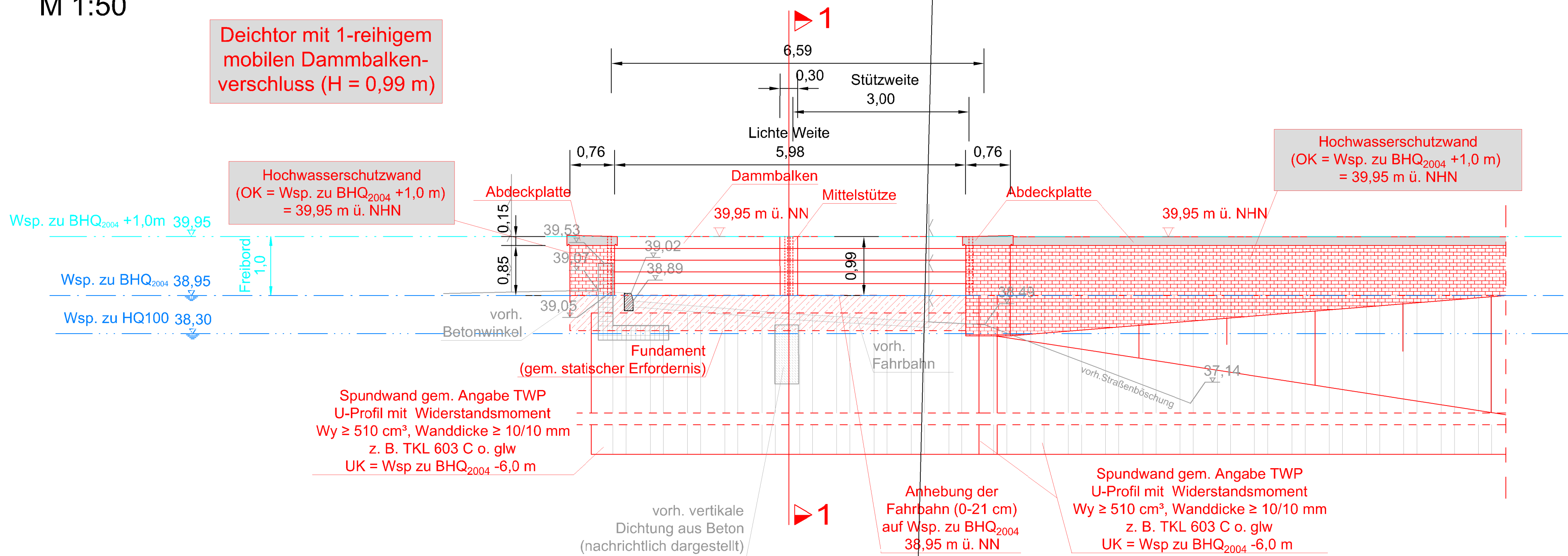
ANSICHT A-A M 1:50
